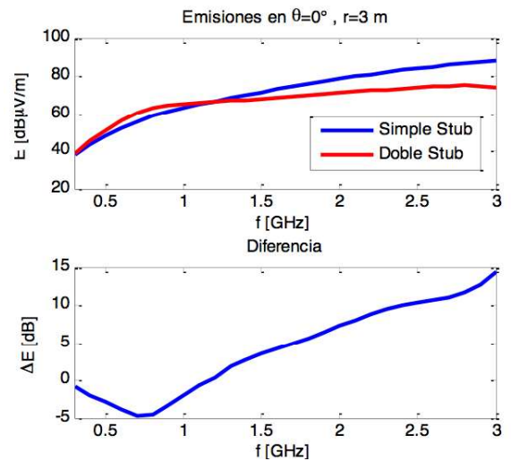
Figura 5. Emisiones del filtro pasabajas (mejor caso)
