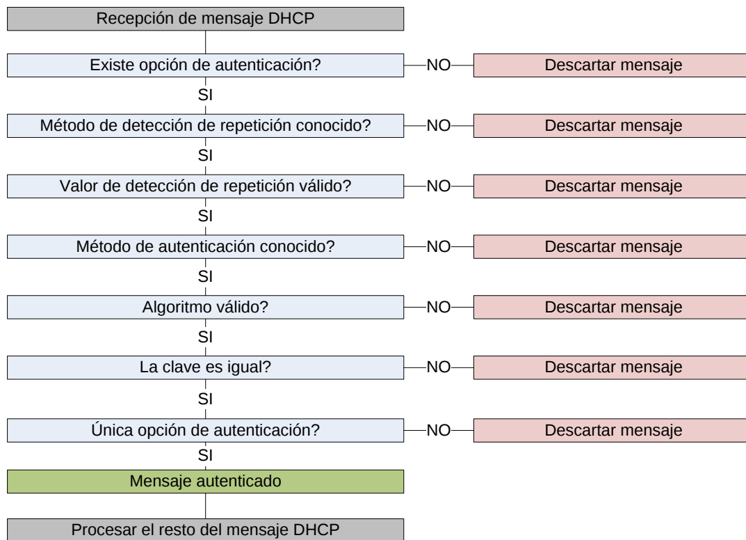
Figura 3.2 Diagrama de flujo de validación de mensajes usando Configuration Token.
