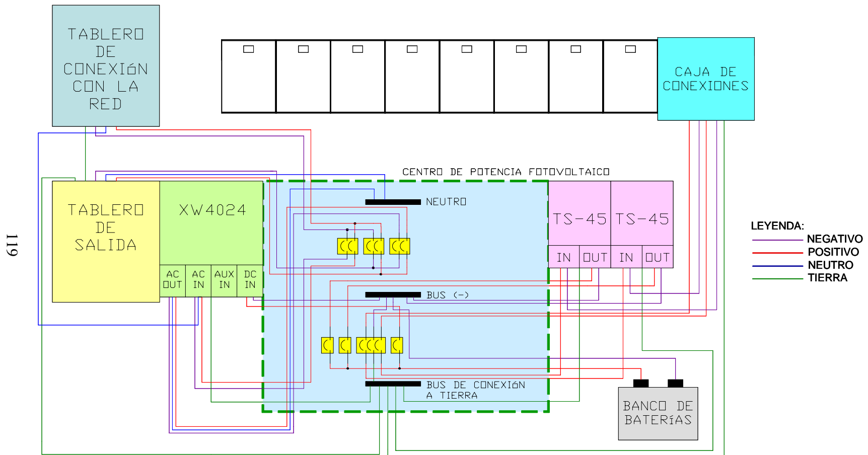
[Anexo 3.3]. Diagrama de conexión del Sistema del Laboratorio de Máquinas Eléctricas
