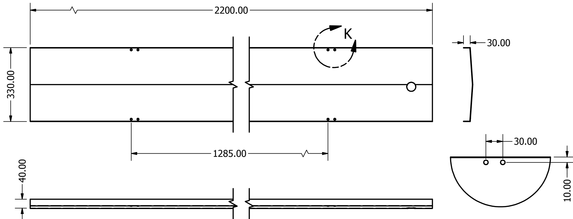
DETALLE K ESCALA 1 / 4
