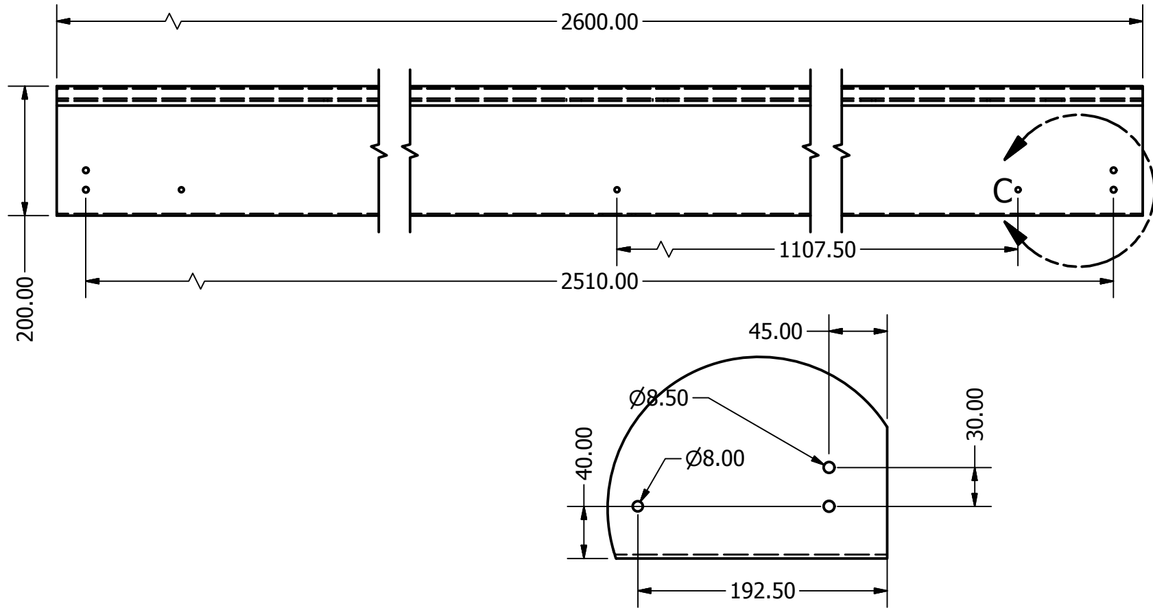
DETALLE C ESCALA 1 / 4
