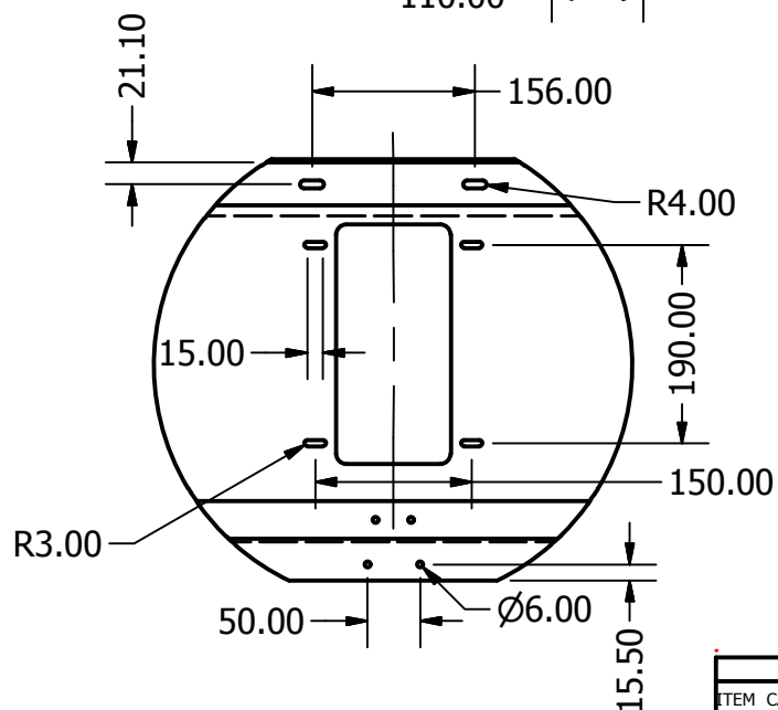
DETALLE A ESCALA 1 : 8
