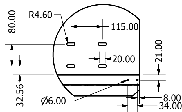
DETALLE B ESCALA 1 / 8
