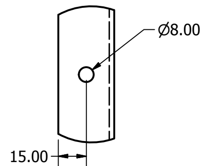
DETALLE L ESCALA 1 : 2
