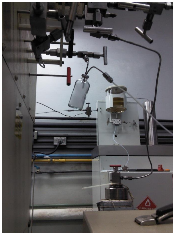
CONTENEDOR DE LÍQUIDO RETROGRADO
