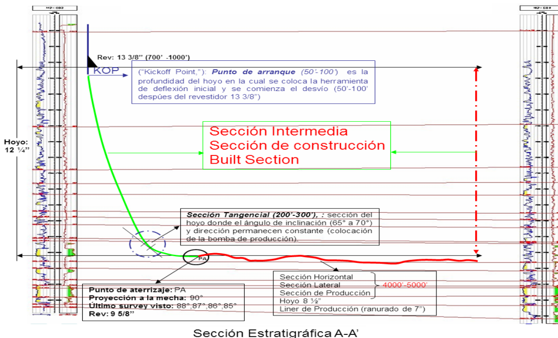
Figura 60 - Conceptos básicos de la perforación direccional (Ronny, 2010) [22]
