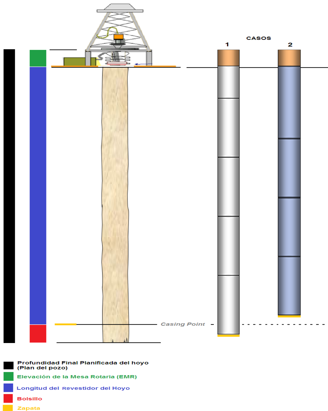
Figura 126 - Esquema de la profundidad final planificada del hoyo [Aristimuño y Briceño, 2012]
