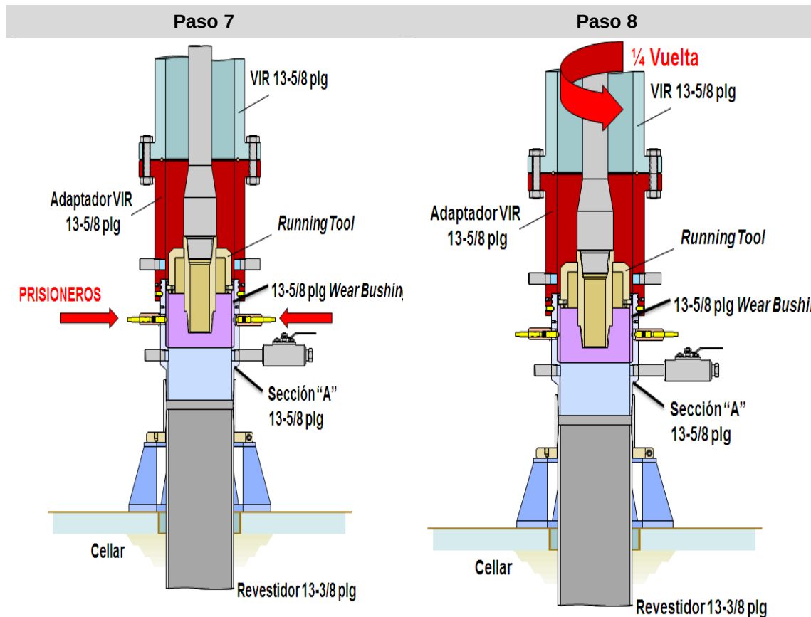
Figura 130 - Secuencia gráfica al insertar el Wear Bushing (Parte II) (Cameron, s.f.) [30]
