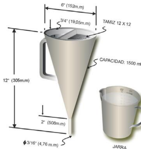
Figura 22 – Embudo Marsh con taza (Prieto, 2007) [13]
