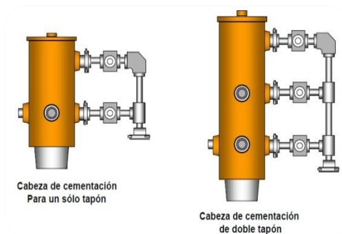
Figura 46 - Cabezal de cementación (Schlumberger, s.f.) [15]
