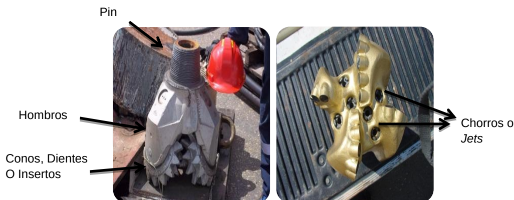
Figura 31 - Partes de la mecha [Aristimuño y Briceño, 2012]
