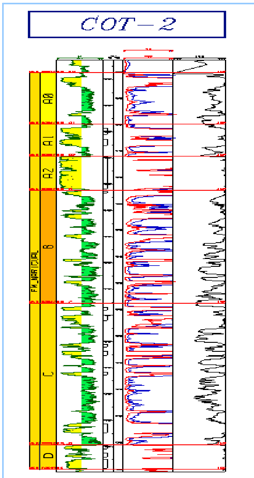
Figura 5.3 Registro tipo del pozo COT-2, definición de topes y bases
