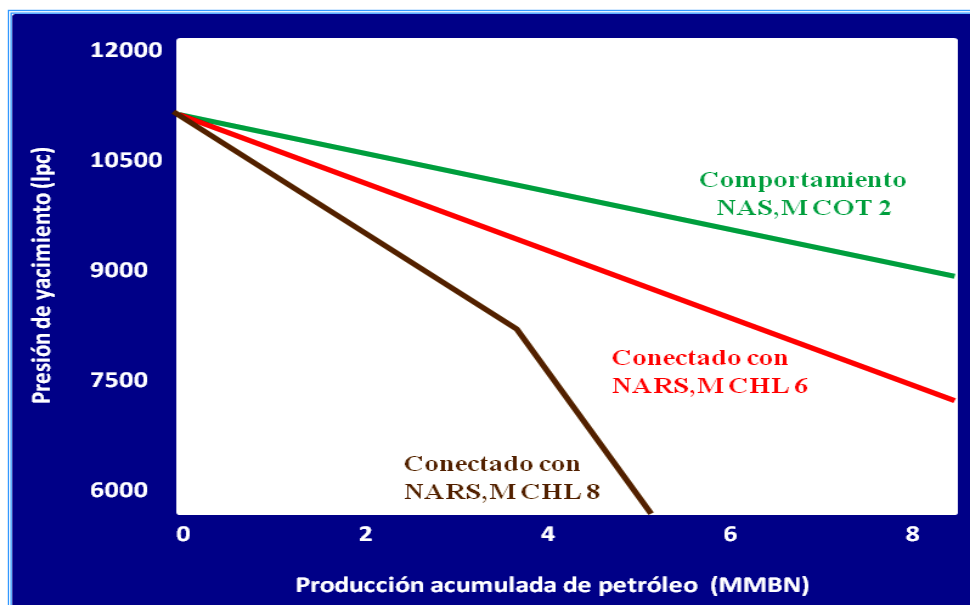
Figura 5.28 Método Analítico del BM, escenarios de estudio
