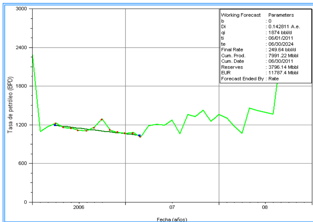
Figura 7-A Comportamiento de producción, período 1
