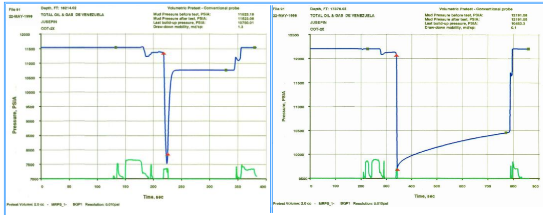
Figura 4.4 Registro MDT. A la izquierda punto de presión estable, a la derecha punto no estabilizado
