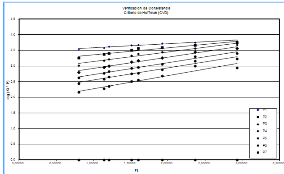
Figura 2.8 Verificación de consistencia, criterio de Hoffman (Martínez, 2009)
