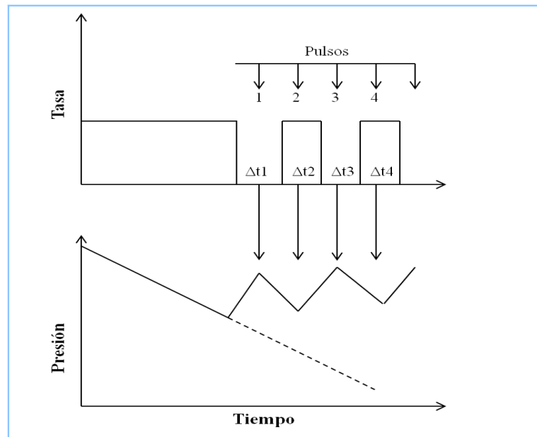
Figura 2.12 Comportamiento de presión en una prueba de pulso (Azuaje, 2011)
