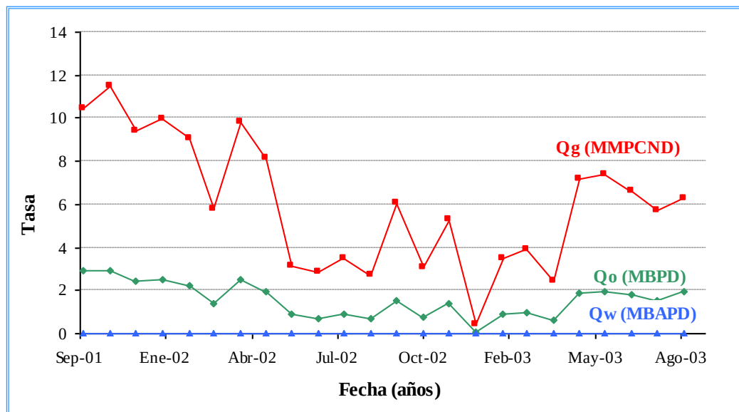
Figura 5.14 Producción Arenas A 1 y A 2 . Desde Septiembre 2001 hasta Agosto 2003
