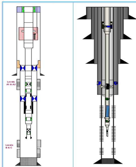
Figura 5.1 Diagrama mecánico del pozo COT-2. A la izquierda el original y a la derecha el generado en este estudio.
