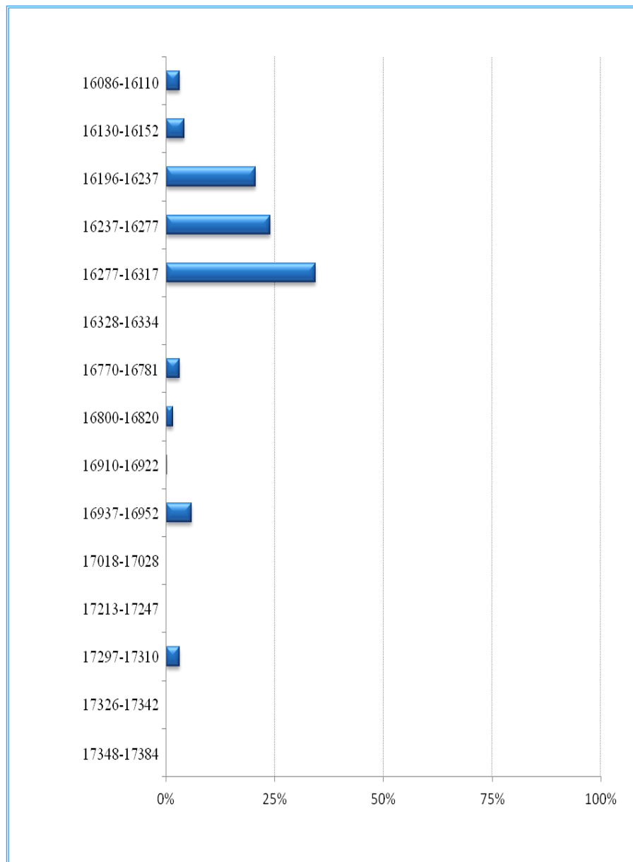
Figura 1-A Perfil de producción inicial pozo COT-2
