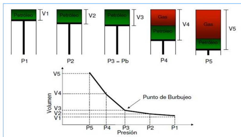
Figura 2.4 Proceso de liberación instantánea (Da Silva, 2010)
