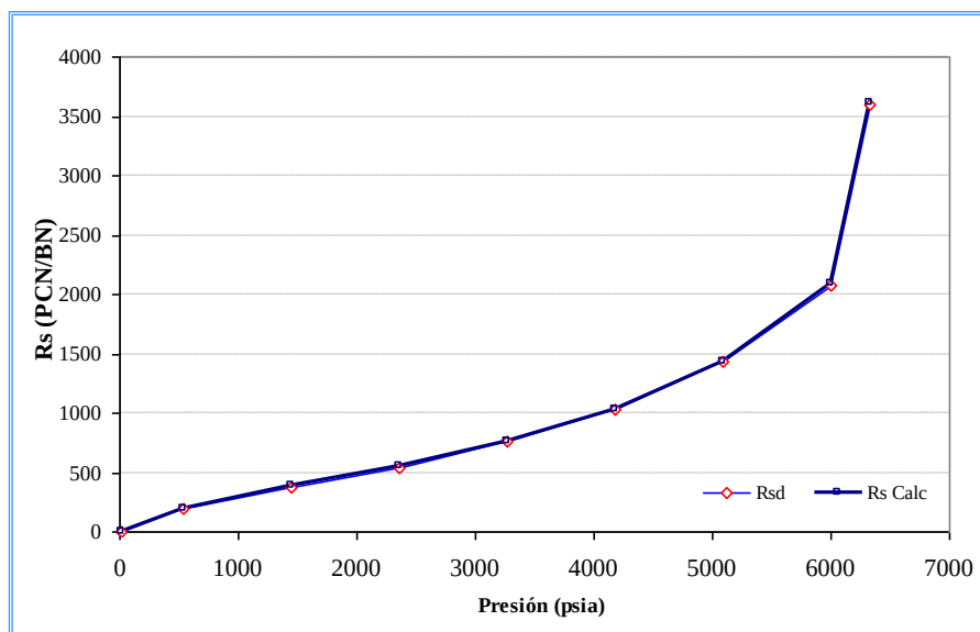
Figura 5-B Gráfica Rs de la prueba y calculado
