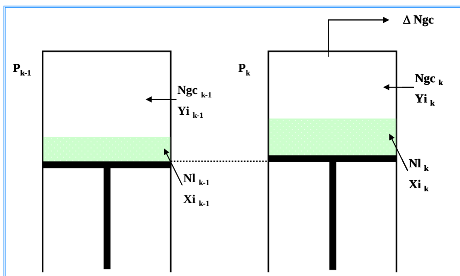
Figura 2.9 Conceptualización de la prueba CVD entre las presiones P_{k-1} y P_k (Modificado de Rojas, 2003)
