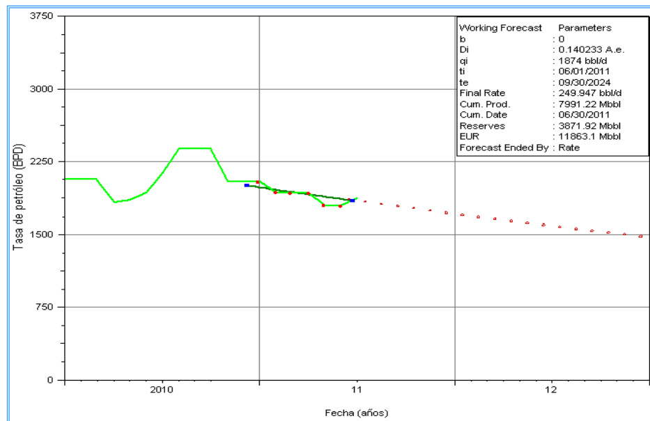
Figura 5.24 Comportamiento de producción, período 4
