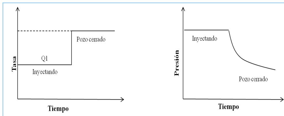
Figura 2. 11 Comportamiento de presión y tasa en una prueba de disipación de presión (Azuaje, 2011)
