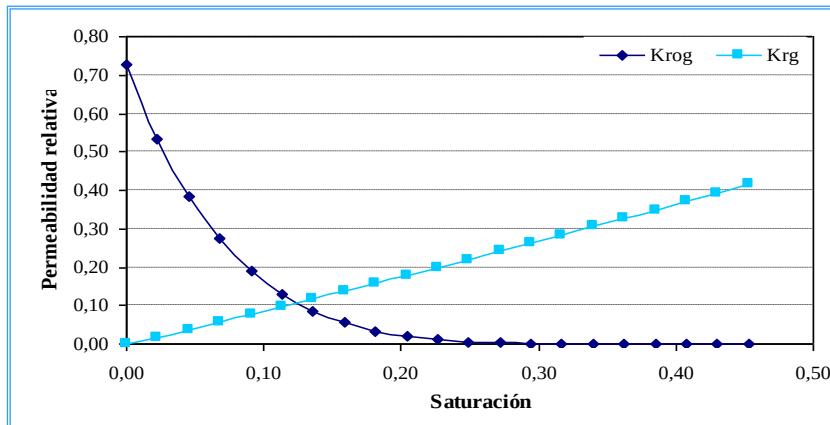
Figura 5.8 Permeabilidades relativas. Sistema Gas-Petróleo
