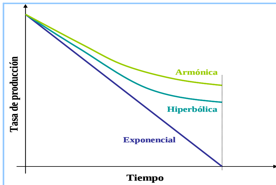
Figura 2.2 Tipos de declinación de producción (Modificado de Barani, F.; Villamil, A., 2005)
