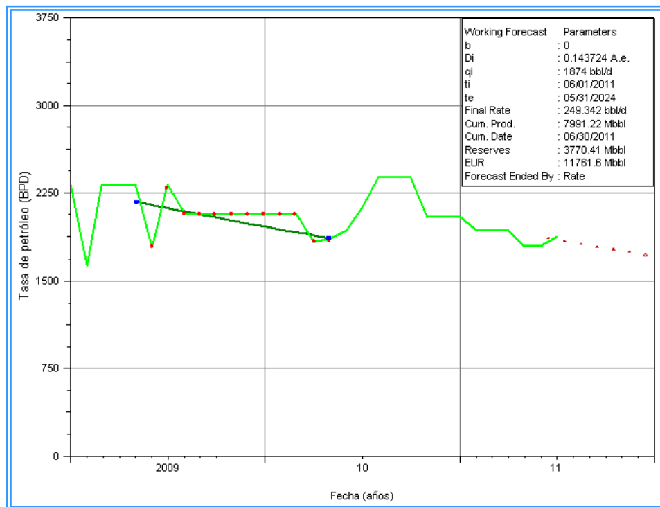
Figura 7-C Comportamiento de producción, período 3
