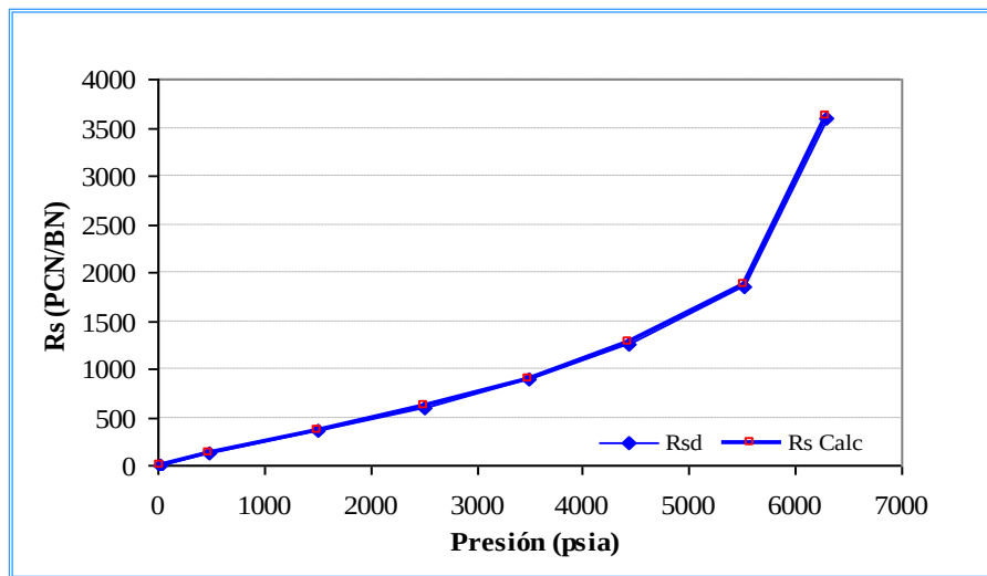
Figura 5.12 Gráfica Rs de la prueba y calculado
