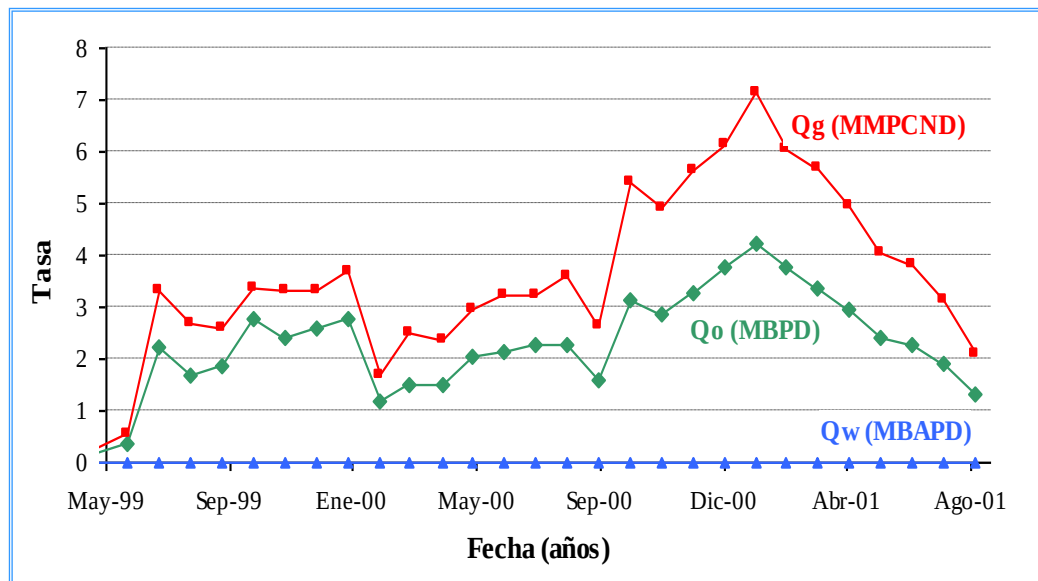
Figura 5.13 Producción Arenas C y D. Desde Mayo 1999 hasta Agosto 2001
