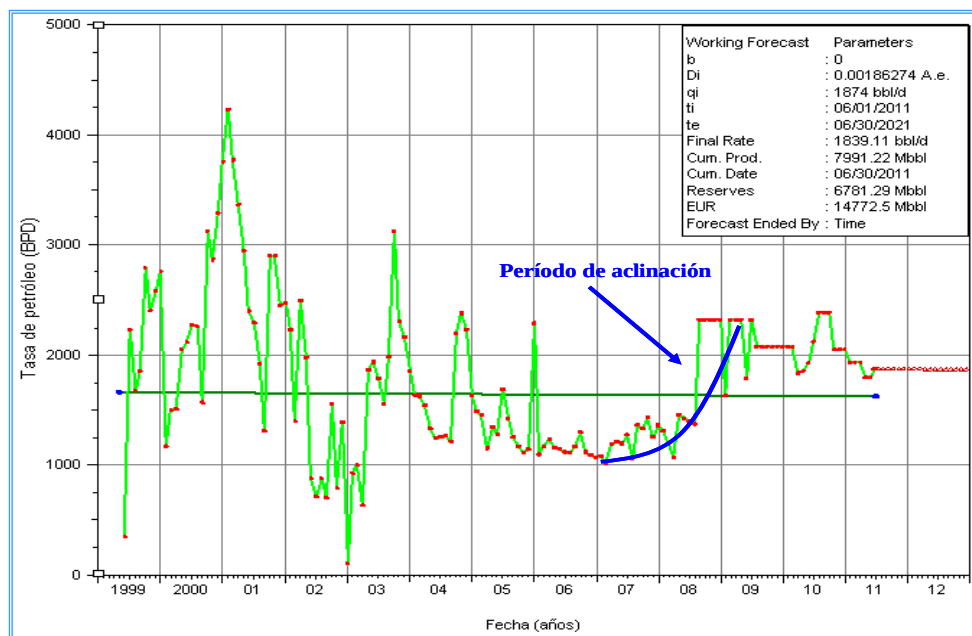
Figura 5.23 Comportamiento de producción del pozo COT-2
