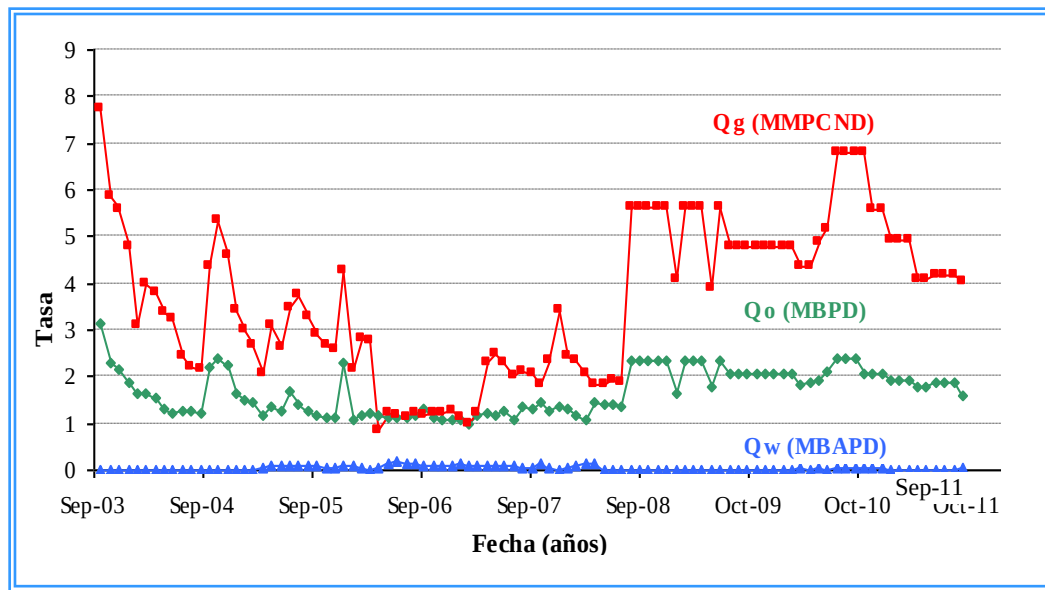
Figura 5.15 Producción Arenas C y D. Desde Septiembre 2003 hasta Septiembre 2011
