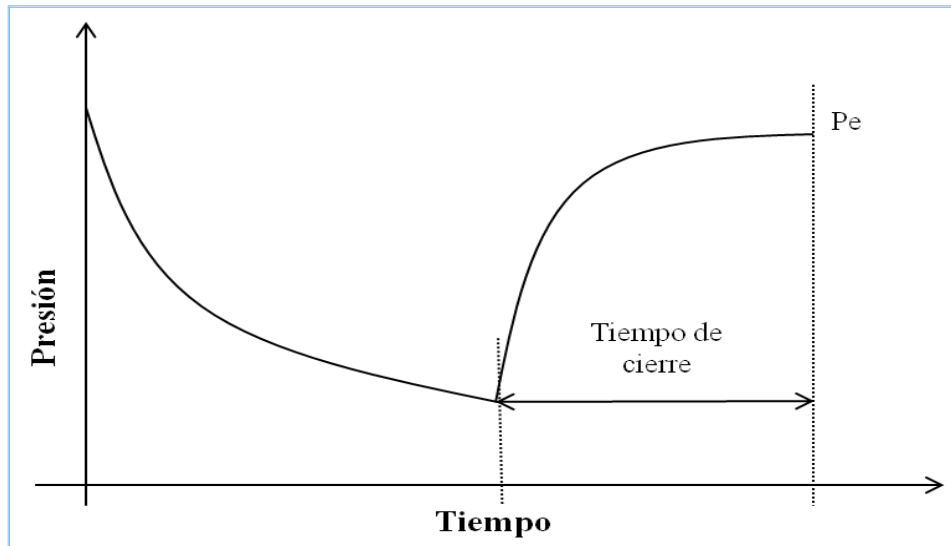
Figura 2.10 Comportamiento de prueba de restauración de presión (Azuaje, 2011)
