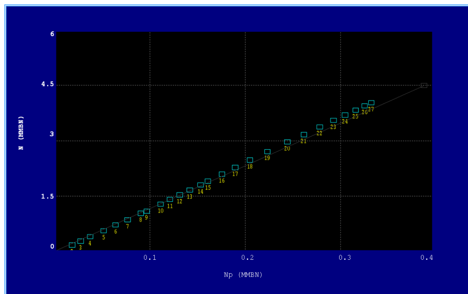
Figura 5.27 Linealización de la EBM
