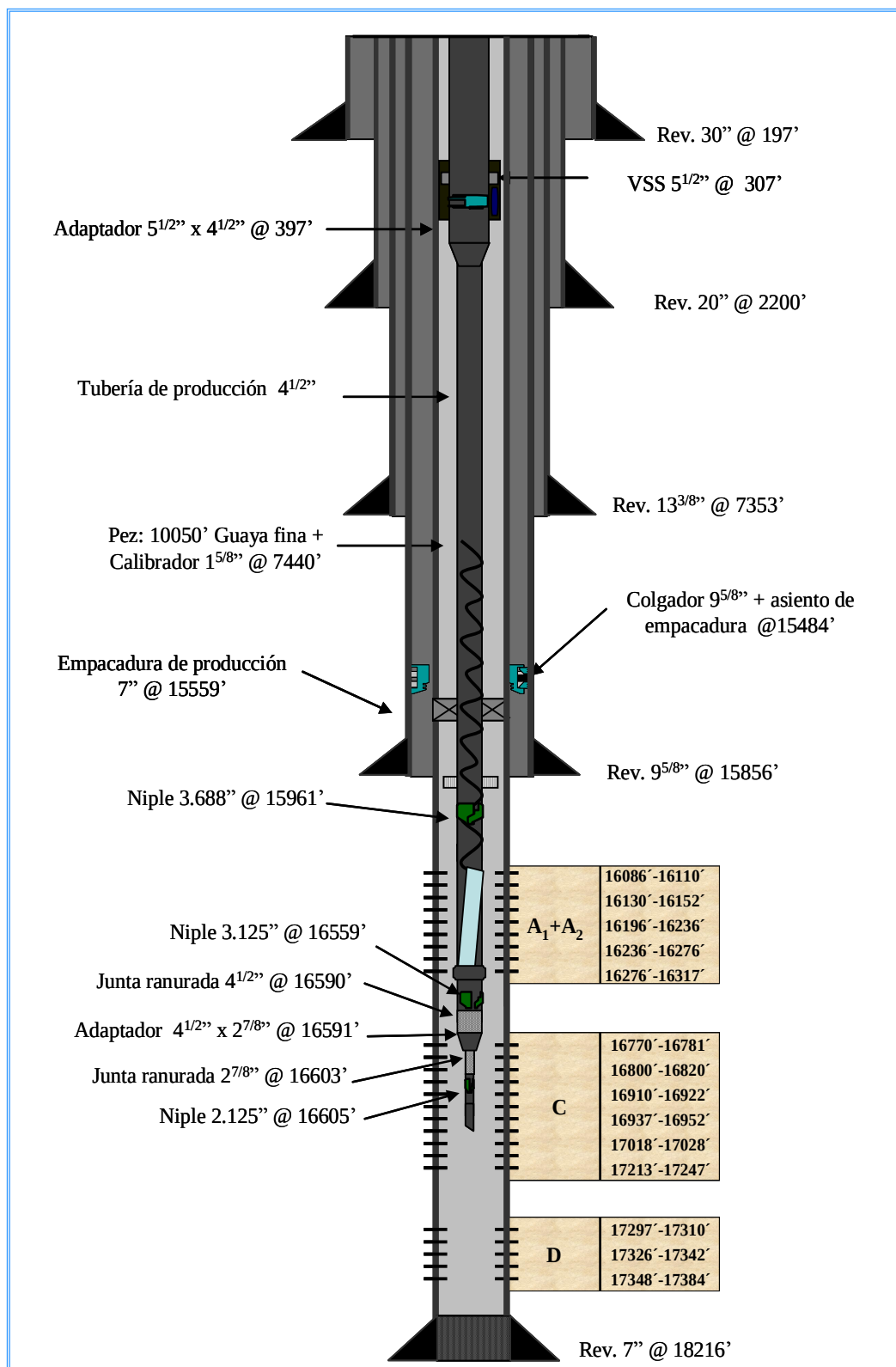
Figura 3-A Diagrama mecánico, pozo COT-2
