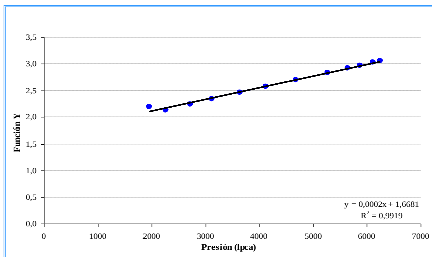
Figura 5.11 Verificación de Función Y
