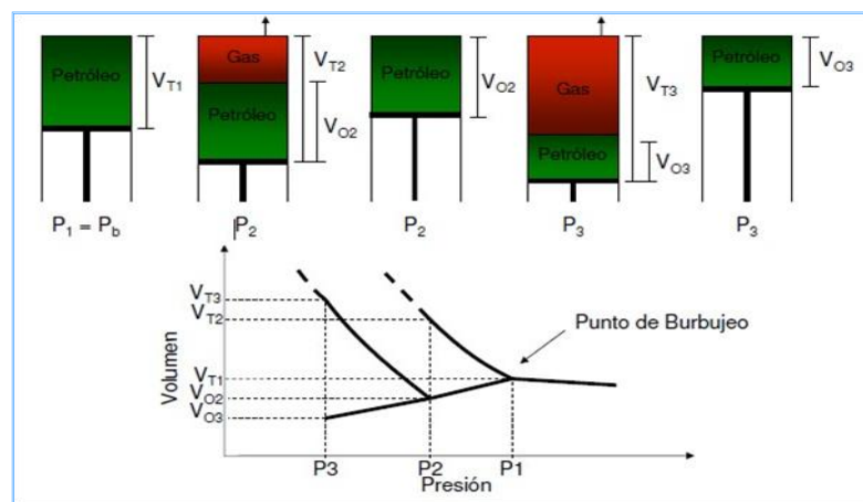
Figura 2.5 Proceso de liberación diferencial (Da Silva, 2010)
