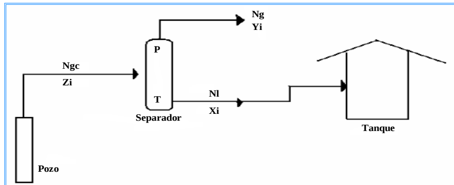
Figura 2.7 Arreglo de separador y tanque de prueba (Modificado de Rojas, 2003)
