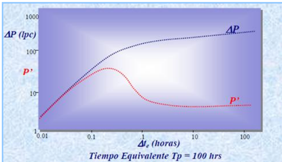
Figura 2.14 Gráfica logarítmica de la Derivada de Bourdet (Salazar, 2011)
