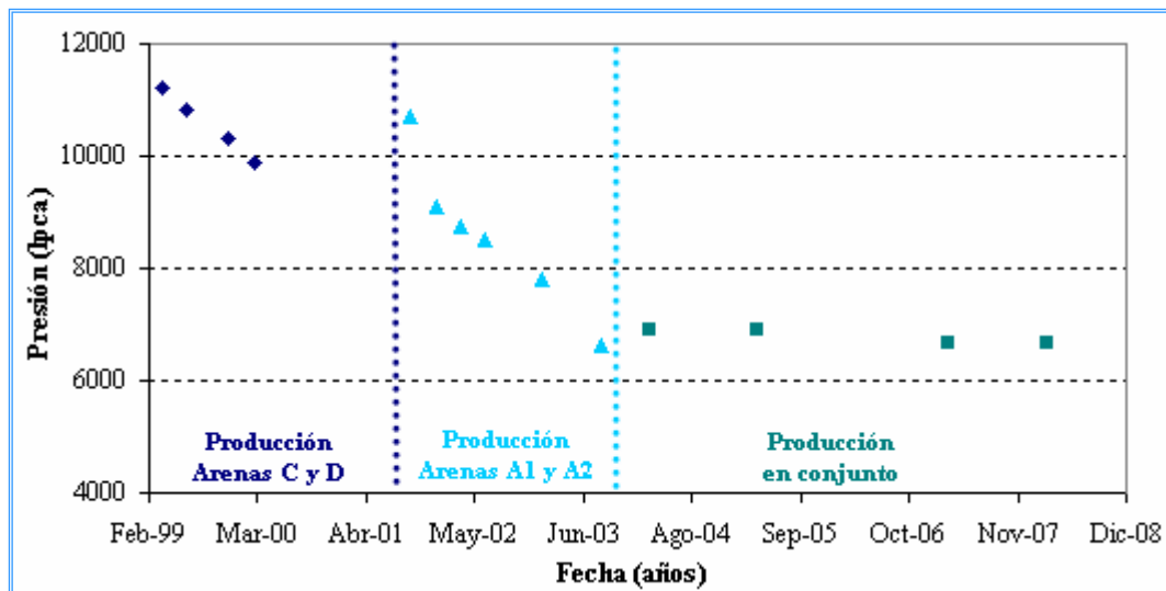
Figura 5.17 Historia de presión del yacimiento respecto al tiempo
