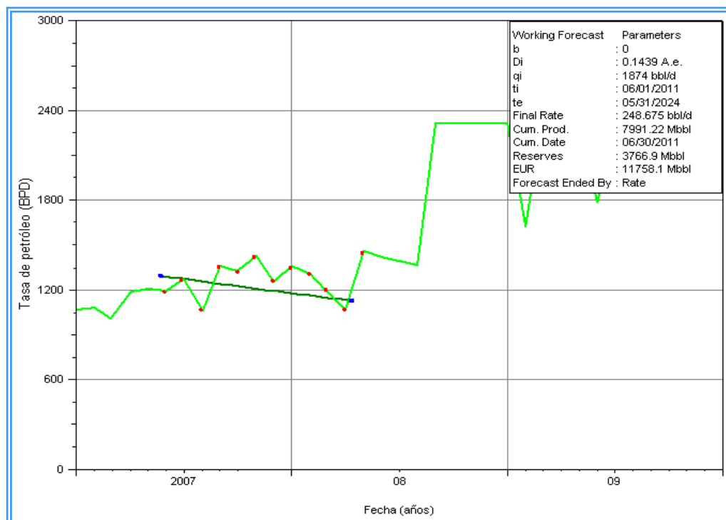
Figura 7-B Comportamiento de producción, período 2
