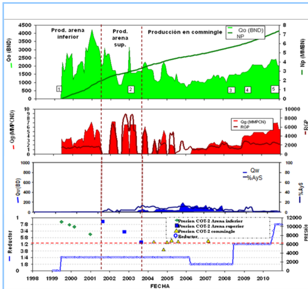
Figura 5.18 Histórico de producción respecto al tiempo
