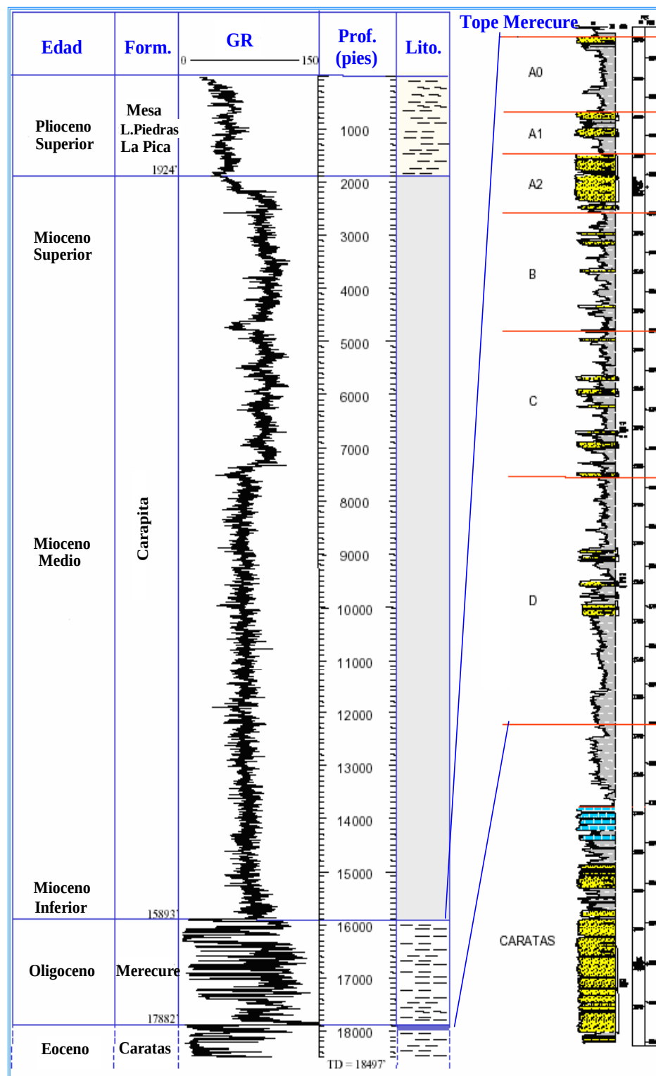
Figura 3.5 Columna estratigráfica típica del Campo Cotoperí (Modificado de Desarrollo de Yacimientos-PDVSA, 2009)
