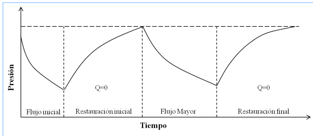
Figura 2.13 Comportamiento de presión en una prueba DST (Azuaje, 2011)
