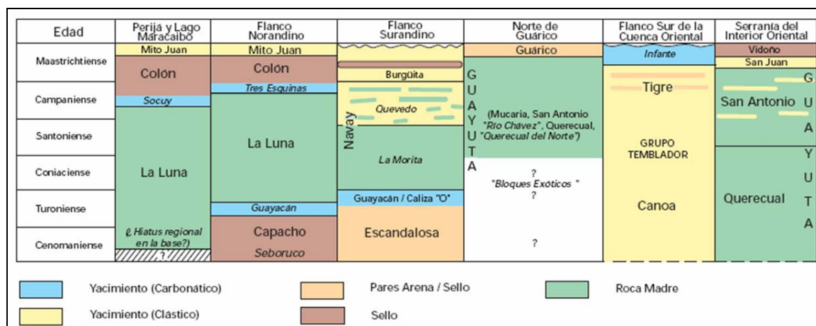
Figura 2.- Cuadro de Correlación Estratigráfica del Cretácico Tardío, donde se observan las formaciones depositadas en este tiempo, en las diversas cuencas geológicas de Venezuela, haciendo énfasis en las rocas madres, productoras y sello, respectivamente. (Tomado y modificado, WEC, 1997)
