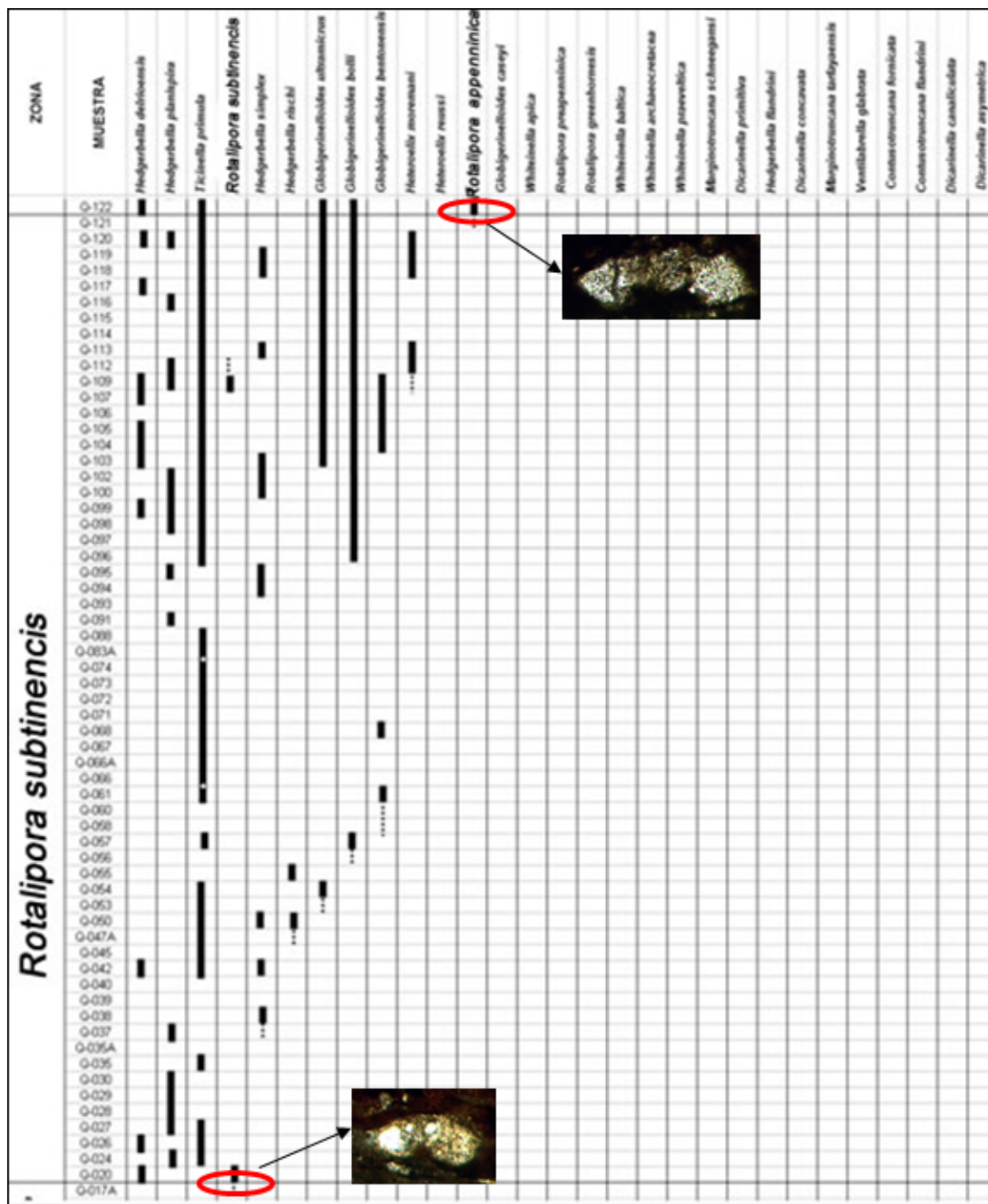
Figura. 36.- Carta cronoestratigráfica de la Subzona Rotalipora subtinensis .
