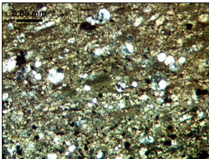
Figura. 15.- Microfacies Mudstone de Foraminíferos Pláncnicos y Radiolarios (MF1). En donde se observa la proporción entre el lodo carbonático (matriz) y las partículas fósiles (pláncnicos y radiolarios). Tomado de Margotta y Ramírez, (2004)
