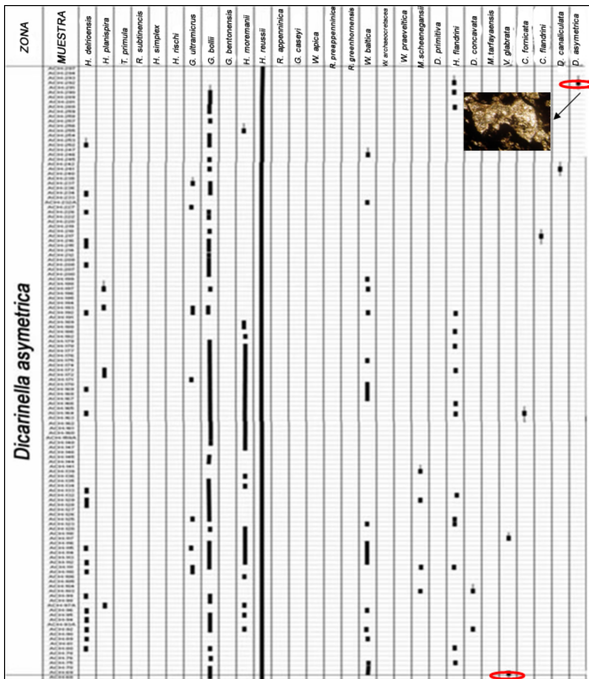
Figura. 42.- Carta cronoestratigráfica representativa de la zona Dicarinella asymetrica .
