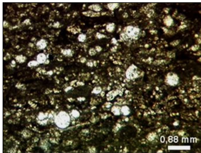
Figura. 17.- Microfacies Wackestone de foraminíferos pláncnicos y radiolarios (MF4). Observándose un mayor porcentaje en las partículas fósiles en matriz con respecto a las 3 MF, anteriores. Tomado de Margotta y Ramírez, (2004)
