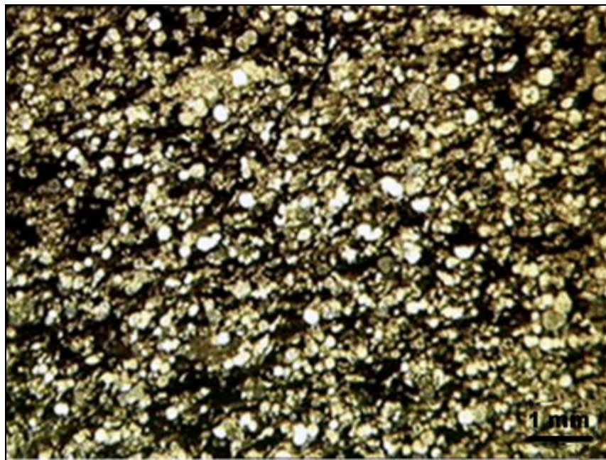
Figura. 19.- Microfacies Packstone de foraminíferos plánticos. (MF8). Obsérvese el alto porcentaje de partículas fósiles con respecto a la matriz.
