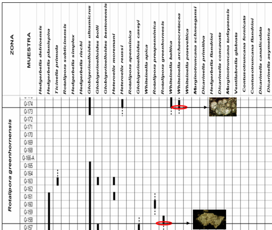
Figura. 38.- Carta cronoestratigráfica, la subzona Rotalipora. greenhornensis .
