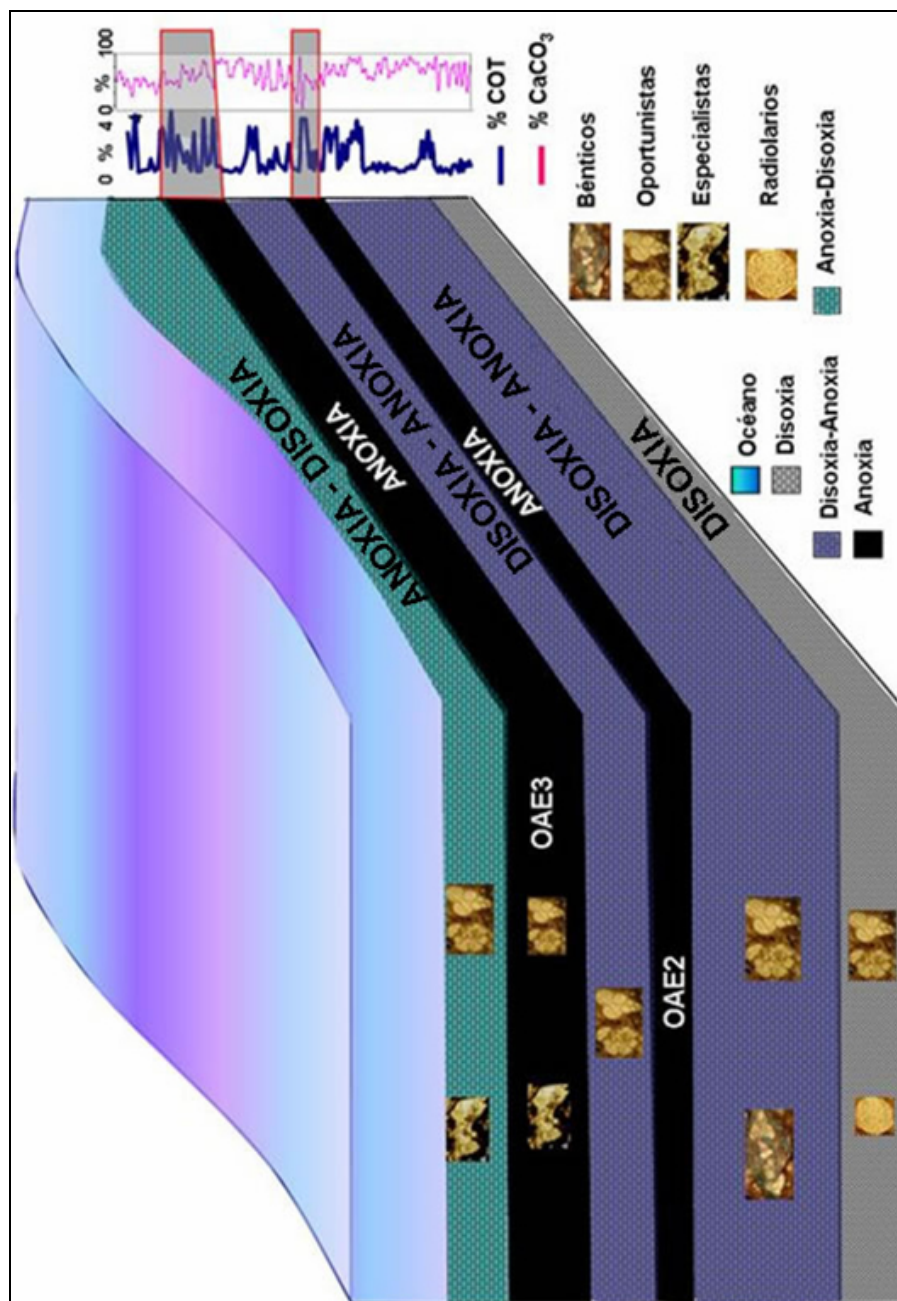
Figura. 55.- Modelo Estratigráfico de la cuenca, en donde se depositó la sección estudiada de la Formación Querecual, localizada en la Isla Chimana Grande. Aquí se observa en detalle las diferentes etapas de anoxia y disoxia ocurrentes, la fauna presente en ella, y las curvas de COT y \text{CaCO}_3 , mostrando sus valores máximos y mínimos respectivamente en los eventos anóxicos, implicando una alta acumulación de materia orgánica, bajos niveles de oxígeno y alta concentraciones de nutrientes necesarios para la supervivencia de los plácticos oportunistas presentes.
