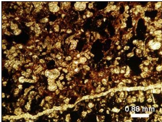
Figura. 18.- Microfacies Wackestone de foraminíferos plácticos. (MF5).
