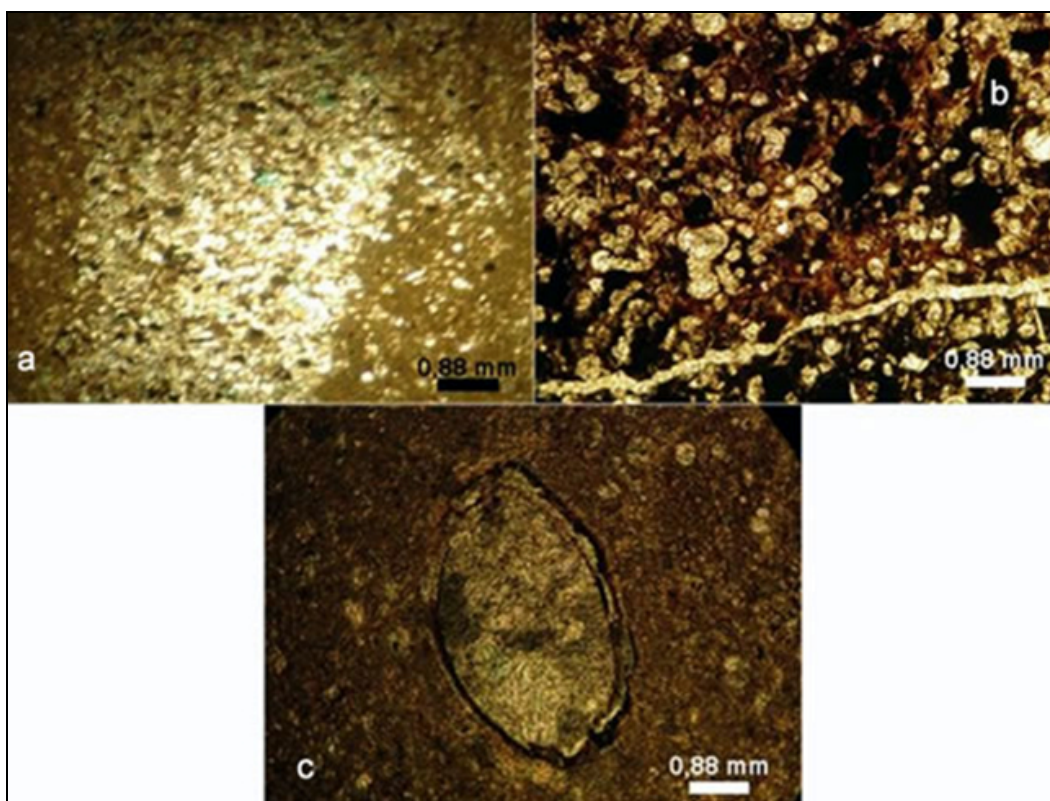
Figura 21.- Presencia de minerales autigénicos cuarzo en matriz (a), pellets de fosfato (b) y calcita relleno un ostracodo (c).
