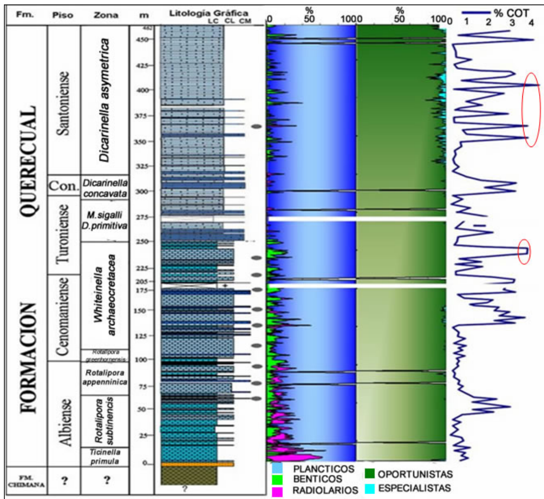
Figura. 50.- Comportamiento del COT, en la Formación Querecual, los valores máximos representan zonas de alta preservación de materia orgánica, estas zonas a su vez presentan un dominio de plánticos oportunistas, lo que indican valores bajos de oxígeno, y alto aporte de nutrientes, evidenciando ciclos de anoxia y disoxia en la cuenca.
