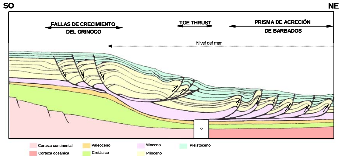
Figura 2.8.- Modelo esquemático costa afuera del Delta del Orinoco y Margen Atlántico de Venezuela, mostrando las complicaciones estructurales mayores (Di Croce, 1995, modificado de Bernardo, 2002)
