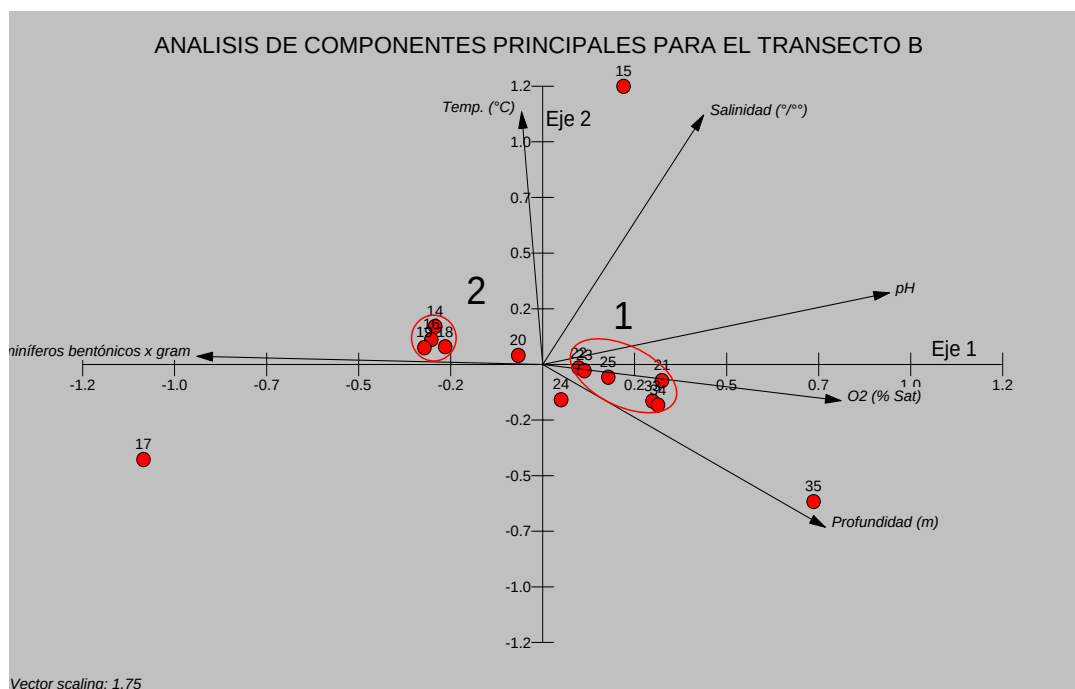
Figura 6.14.- Grafico de análisis de componentes principales para el transecto B
