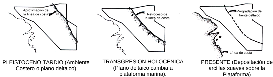
Figura 4.5.- Ambientes depositacionales inferidos (modificado de Mahmood, 1980)
