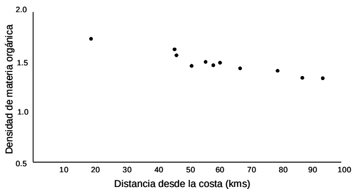
Figura 4.8.- Disminución de la densidad de materia orgánica con la distancia de la costa del Delta del Orinoco (modificado de Nwachukwu y Barker, 1985)
