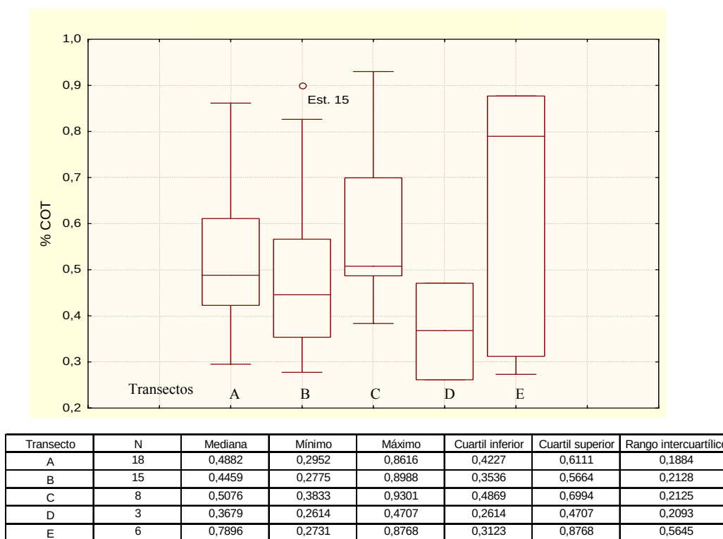
Figura 6.9.- Diagrama de caja gráfica de los valores obtenidos de carbono orgánico total (COT) y resumen de los resultados estadísticos correspondientes a este parámetro.
