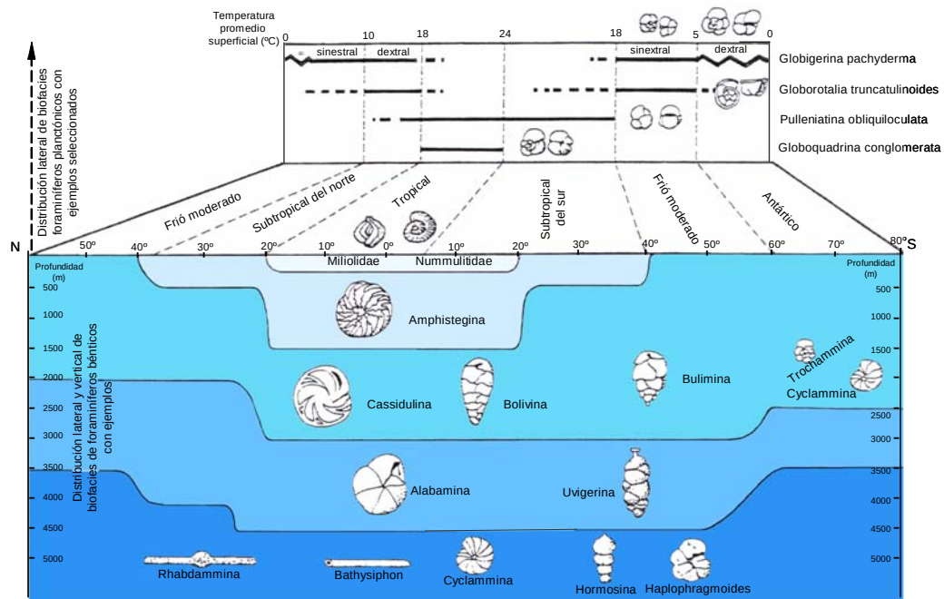
Figura 3.3.- Diagrama ilustrativo de cómo los conjuntos de foraminíferos bentónicos y planctónicos cambian con la profundidad y latitud en el océano Pacífico, especialmente en relación con la temperatura (modificado de Cied, 1998).
