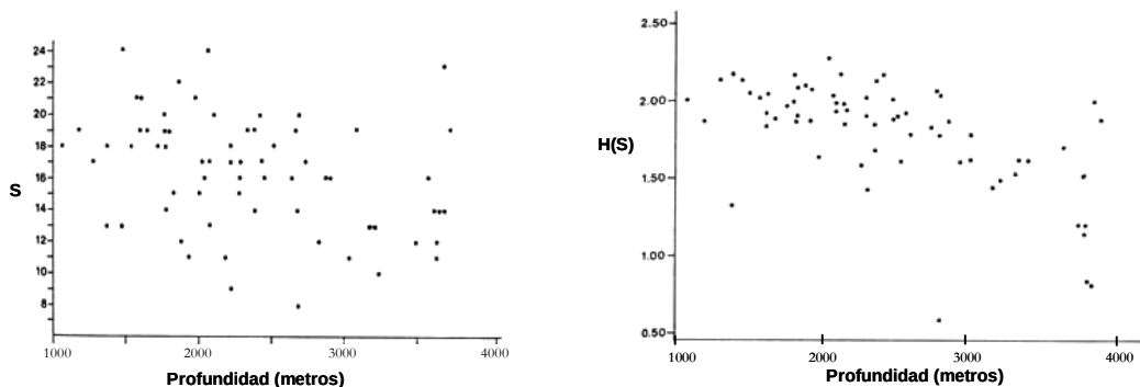
Figura 7.1.- Diversidad de especies de foraminíferos bentónicos del centro del océano Ártico (modificado de Lagoe, 1976).
