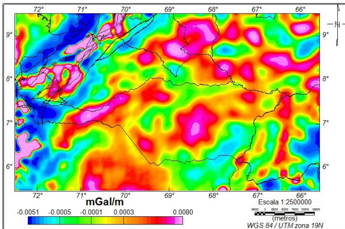
Figura 4.14: Primera derivada en el eje z de la Anomalía de Bouguer.
