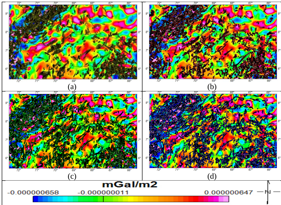
Figura 4.18: Deconvolución de Euler con índice estructural de 3 sobre el mapa de segunda derivada de Anomalía de Bouguer. (a) Soluciones de 0 a 12 km, (b) soluciones de 12 y 15 km, (c) soluciones de 15 a 18 km y (d) soluciones de 18 a 20 km de profundidad.
