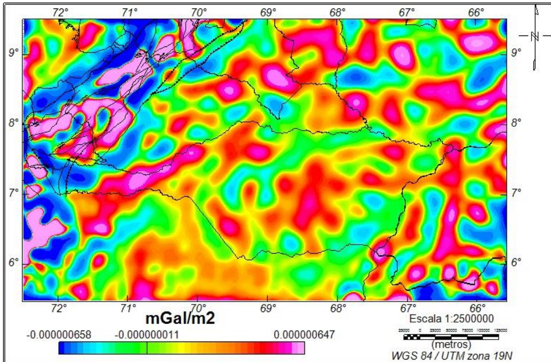
Figura 4.15: Segunda derivada en el eje z de la Anomalía de Bouguer.
