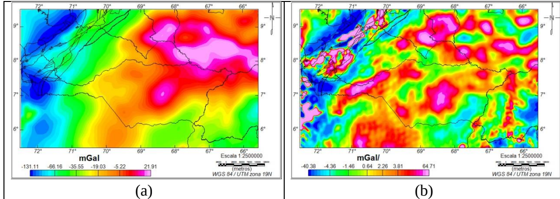
Figura 3.9. Mapas de separación Regional-Residual por continuación analítica del campo de la Anomalía de Bouguer a una altura de 9000 m. (a) mapa regional, (b) mapa residual.
