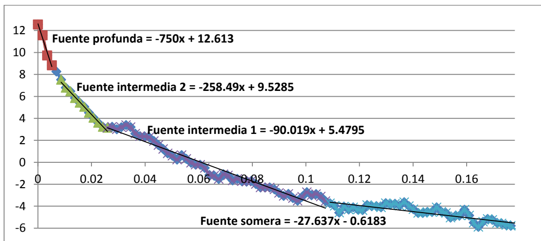
Figura 4.6: Análisis del espectro de potencia.
