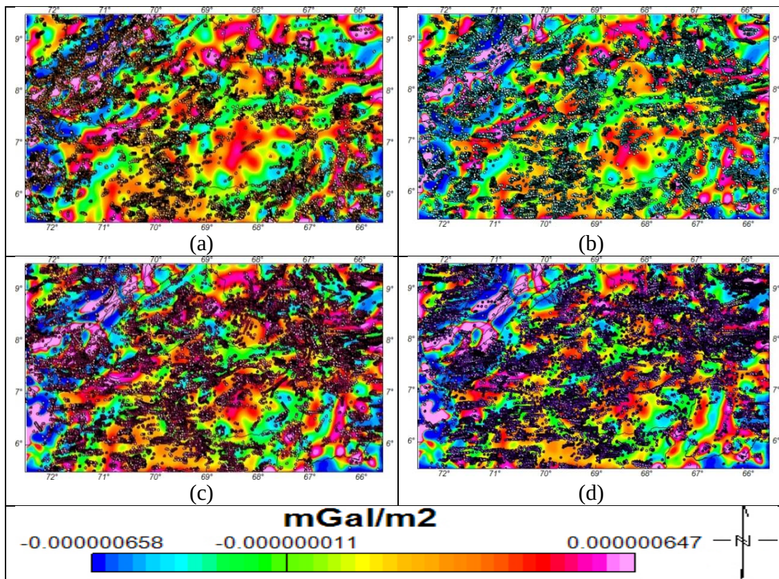
Figura 4.19: Deconvolución de Euler con un índice estructural 3 sobre el mapa de segunda derivada de Anomalía de Bouguer. (a) Soluciones de 20 a 25 km, (b) soluciones de 25 y 30 km, (c) soluciones de 30 a 35 km y (d) soluciones de 35 a 40 km de profundidad.
