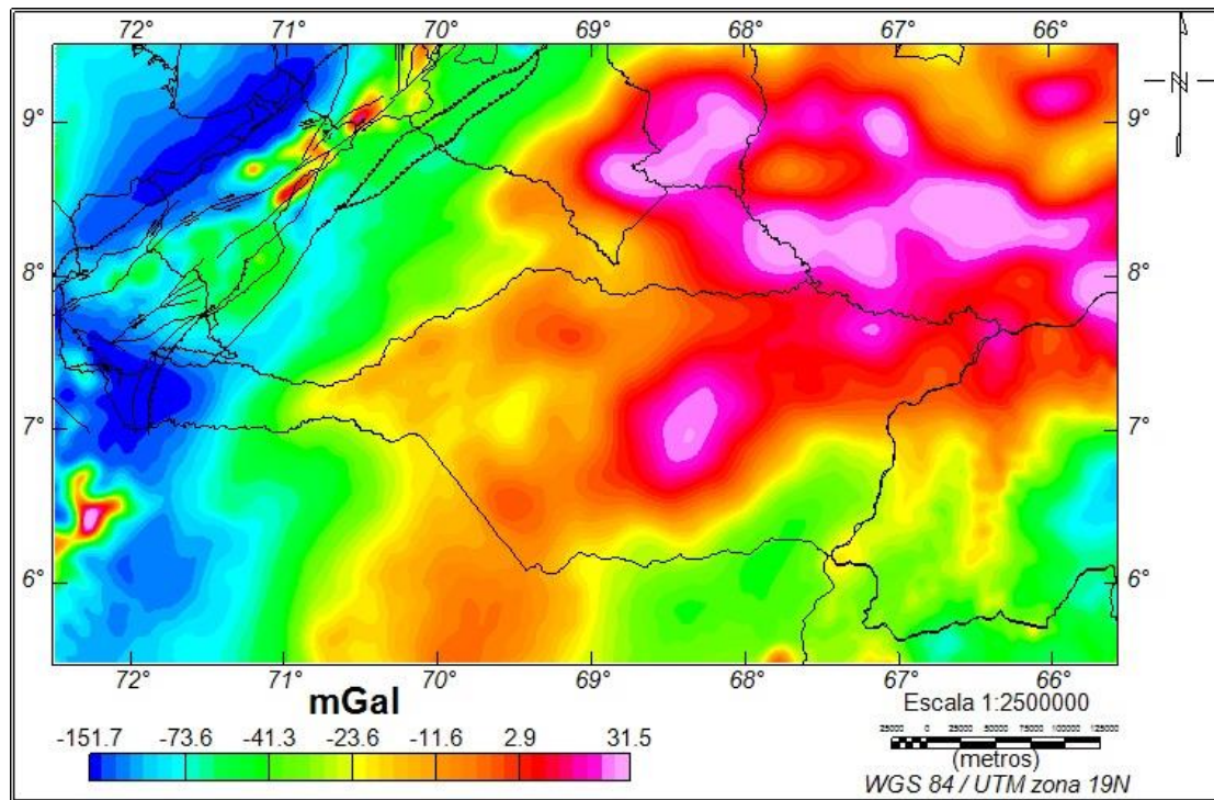
Figura 4.3: Mapa de Anomalía de Bouguer, para una densidad de 2.67 g/ml.
