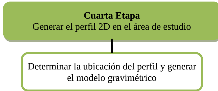
Figura 3.17. Diagrama de flujo sobre la metodología a seguir para generar el perfil 2D en el área de estudio.
