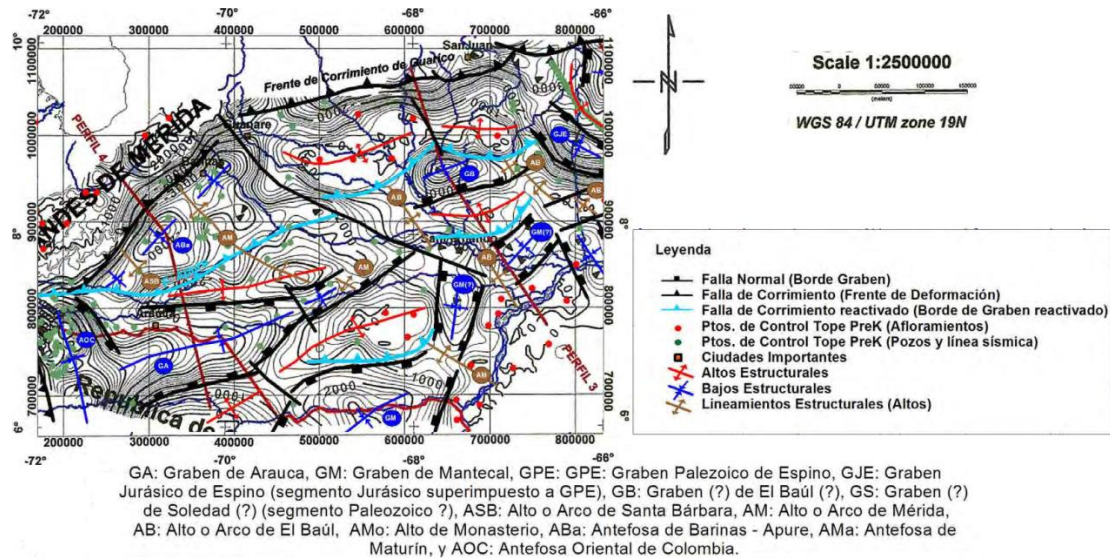
Figura 3.3. Interpretación estructural Basamento pre-K. Tomado y modificado de González (2009).
