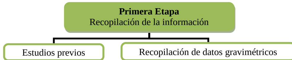
Figura 3.1. Diagrama de flujo sobre la metodología a seguir para la recopilación de información.
