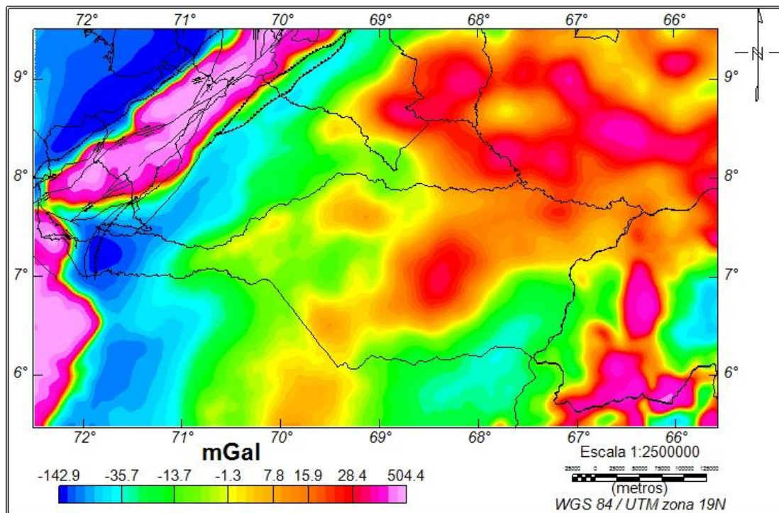
Figura 4.2: Mapa de Anomalía de Aire Libre.
