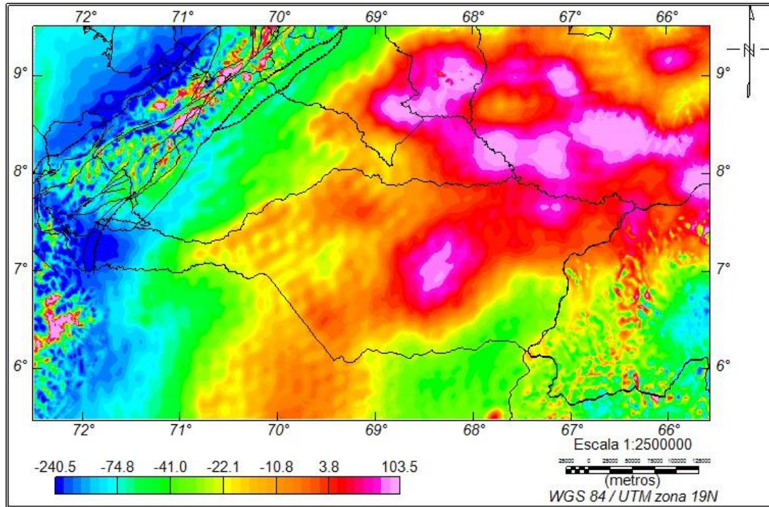
Figura 3.8. Mapa de Anomalía de Bouguer para una densidad de 2.67 g/ml.
