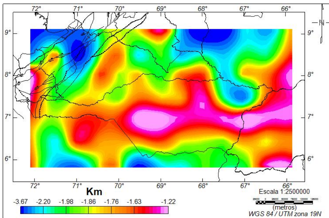
Figura 4.9: Mapa generado a partir de las profundidades someras obtenidas en el análisis espectral.
