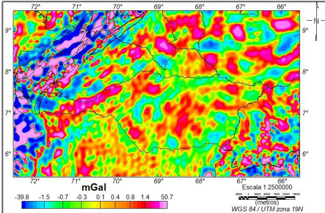
Figura 4.13: Mapa de Anomalía de Bouguer residual.
