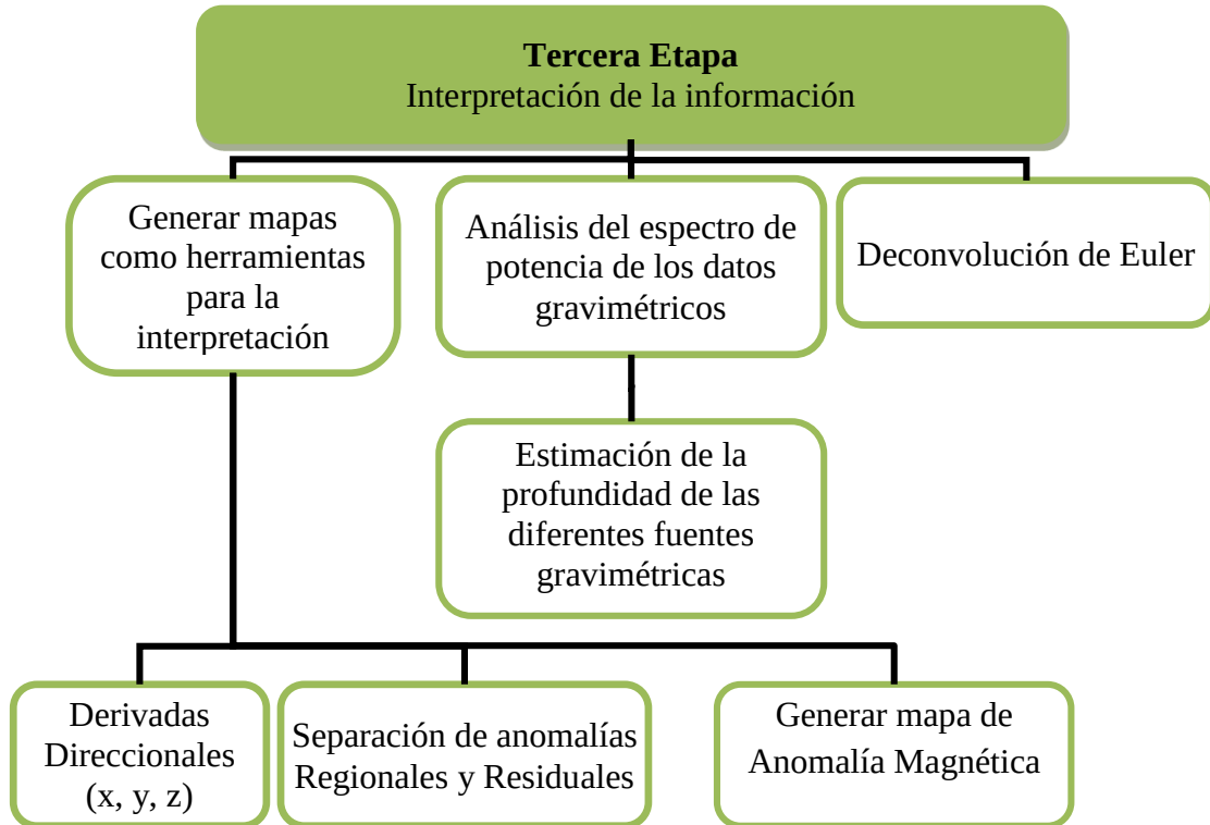
Figura 3.7. Diagrama de flujo sobre la metodología a seguir para la interpretación de la información.
