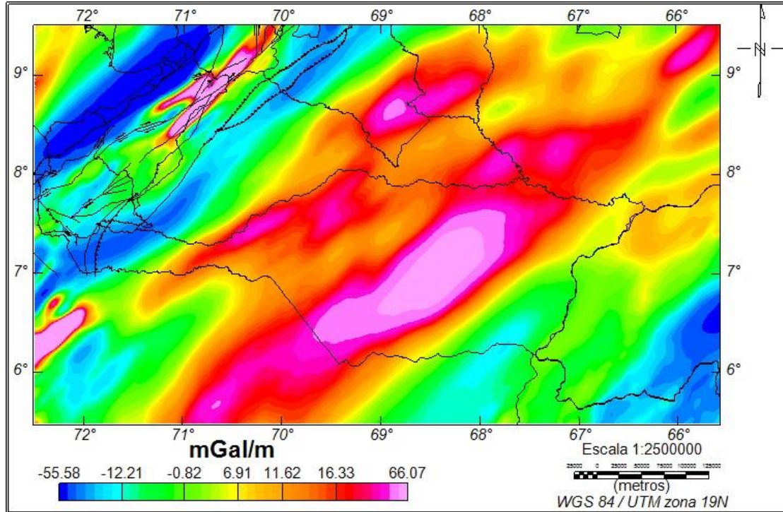
Figura 4.16: Mapa de coseno direccional de 45° de la Anomalía de Bouguer.
