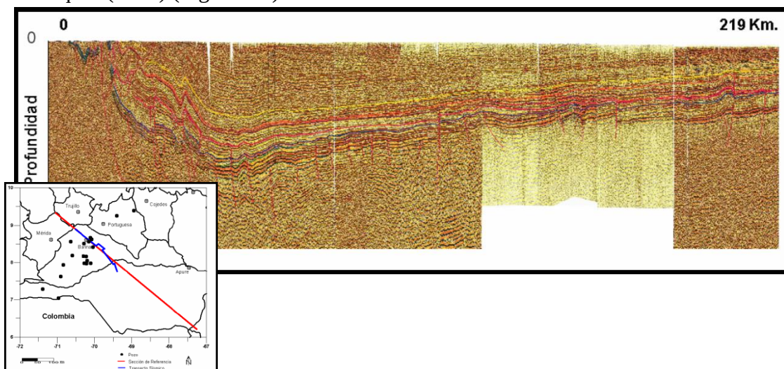
Figura 3.2. Transecto sísmico del estado Barinas (línea azul). Tomado de Henriques (2004).
