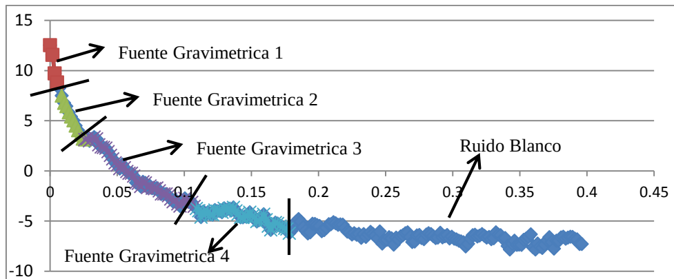
Figura 4.5: Espectro de potencia de los datos de AB.
