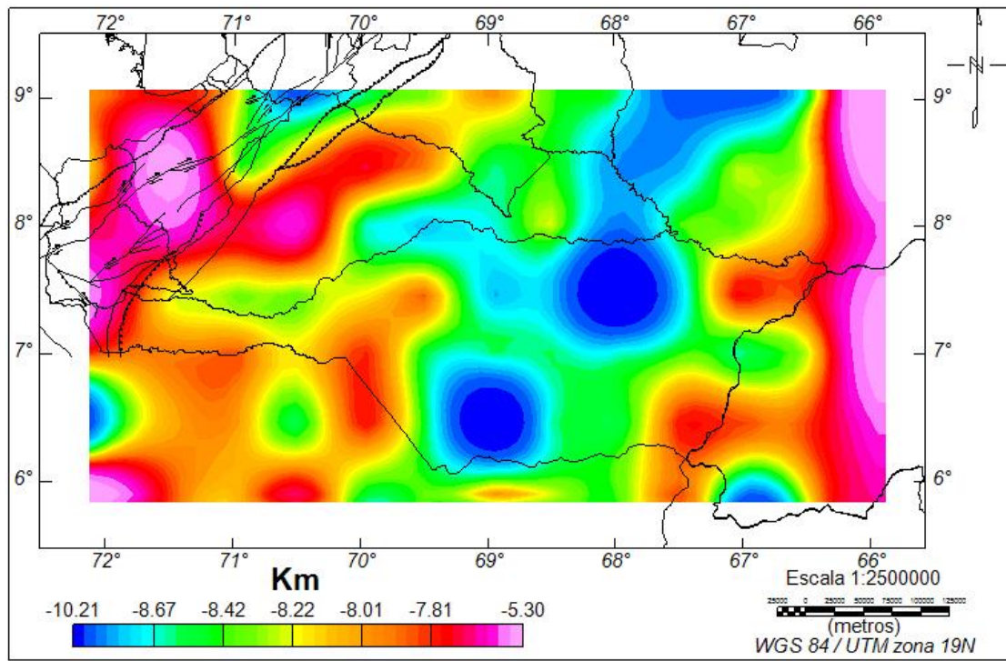
Figura 4.10: Mapa generado a partir de las profundidades intermedia 1 obtenidas en el análisis espectral.
