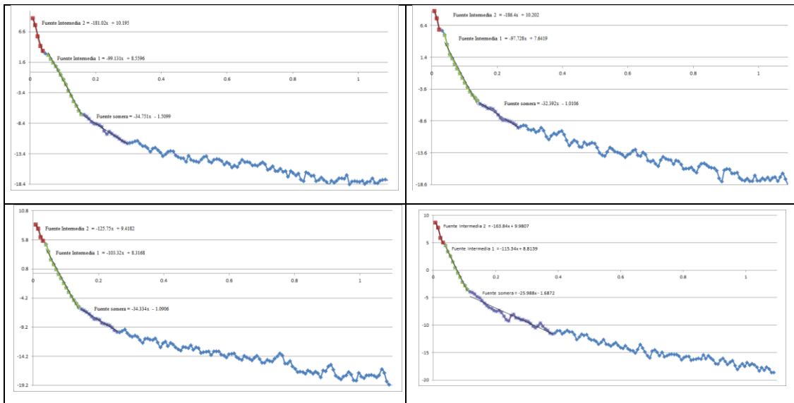
Figura 4.8: Ejemplos del espectro de potencia realizado para cada ventana.
