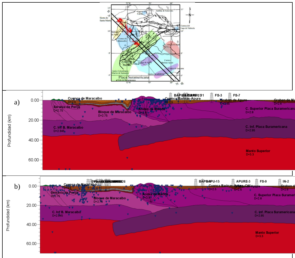
Figura 3.4. Modelos gravimétricos estructurales de la zona noroccidental de Venezuela a) Perfil A-A', b) Perfil B-B'. Tomado y modificado de Arnaiz (2011).
