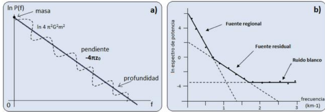
Figura 3.16. a) Representación gráfica del logaritmo neperiano del espectro de potencia respecto a la frecuencia. b) Representación ideal del espectro de potencia frente a la frecuencia. Tomado de González (2014).
