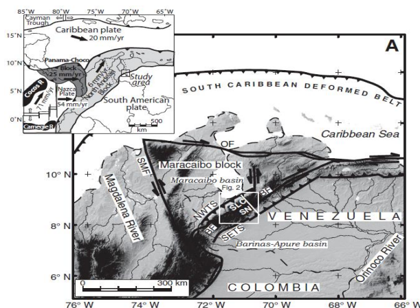
Figura 2.1. Mapa estructural simplificado de los Andes Venezolanos mostrando las fallas rumbo deslizantes más importantes. Modificado de Bermúdez (2011).
