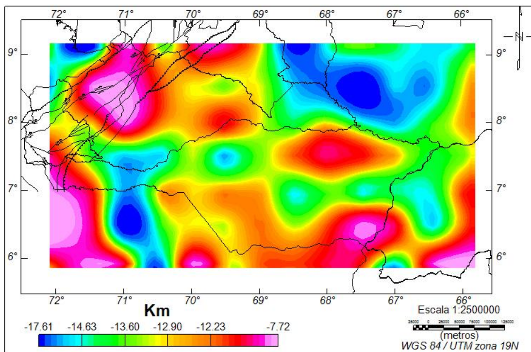
Figura 4.11: Mapa generado a partir de las profundidades intermedia 2 obtenidas en el análisis espectral.
