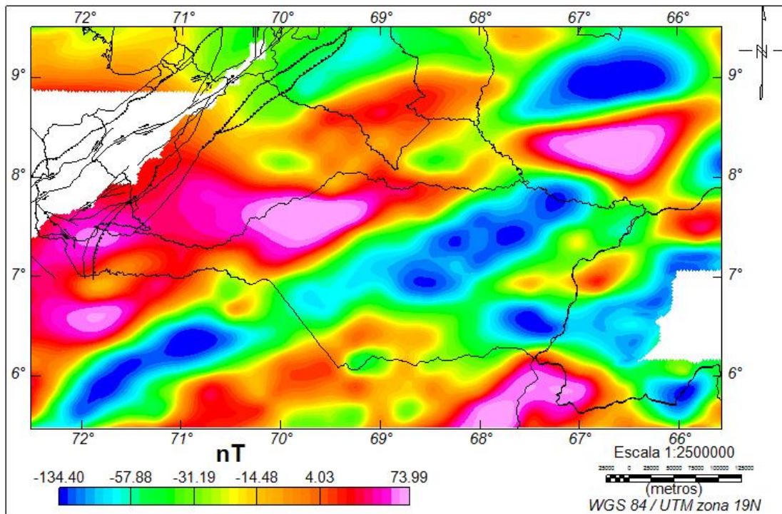
Figura 4.20: Mapa de Anomalía Magnética con reducción al Ecuador.
