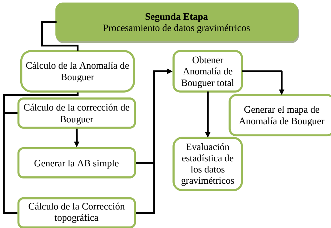
Figura 3.5. Diagrama de flujo sobre la metodología a seguir para el procesamiento de datos gravimétricos.
