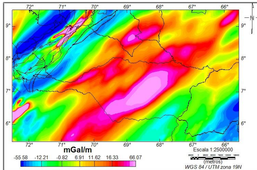
Figura 3.13. Mapa de coseno direccional a un Angulo de 45° de la Anomalía de Bouguer.
