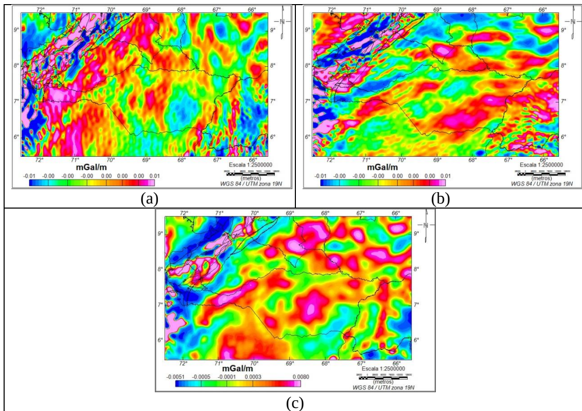
Figura 3.12. Mapas de derivadas direccionales de la Anomalía de Bouguer. (a) derivada en X, (b) derivada en Y, (c) derivada en Z.
