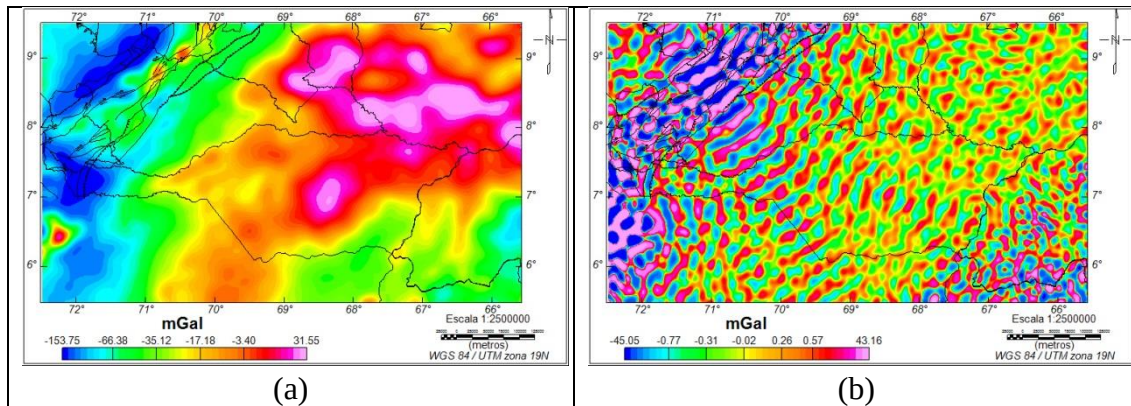
Figura 3.10. Mapas de separación Regional-Residual por filtro pasa banda de la Anomalía de Bouguer a una frecuencia de corte de 0.026. (a) mapa regional, (b) mapa residual.
