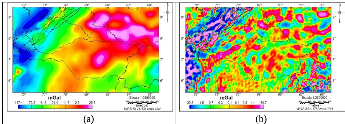
Figura 3.11. Mapas de separación Regional-Residual por filtro gaussiano de la Anomalía de Bouguer a una frecuencia de corte de 0.026. (a) mapa regional, (b) mapa residual.
