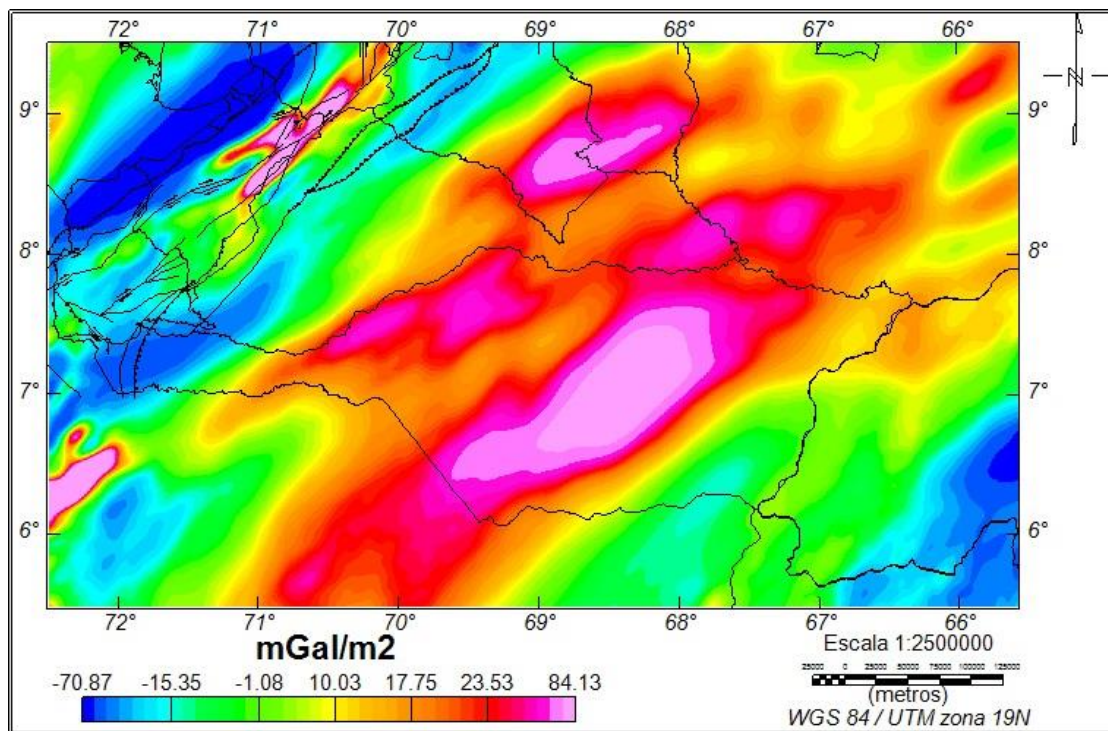
Figura 4.17: Mapa de coseno 2 direccional de 45° de la Anomalía de Bouguer.
