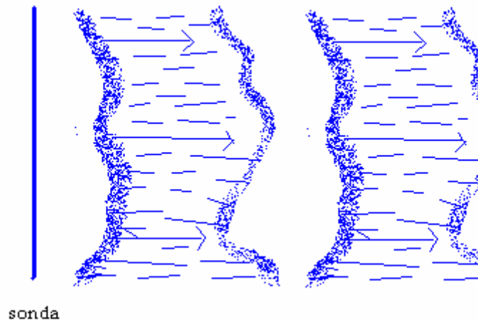
Figura 3.2: Flujo laminar de agua, a través de un medio poroso.
