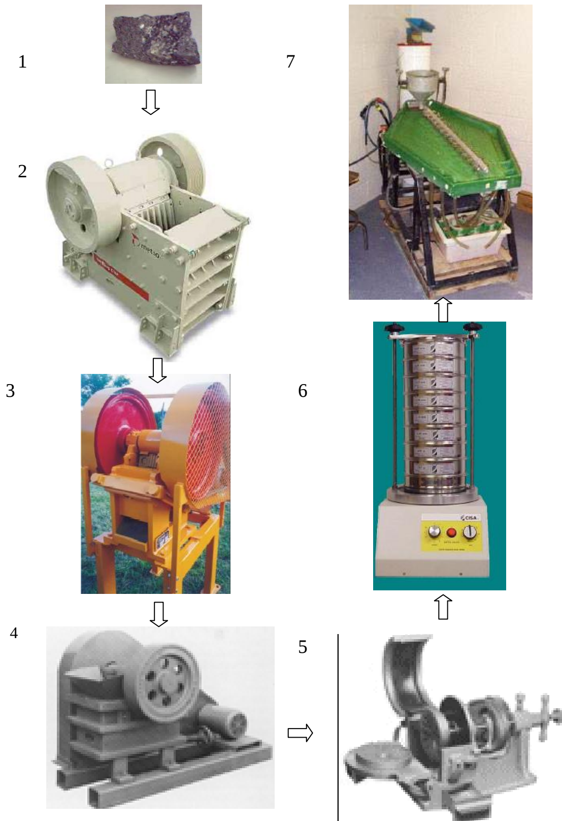
Figura 3.5: Esquema convencional para la concentración de minerales pesados
