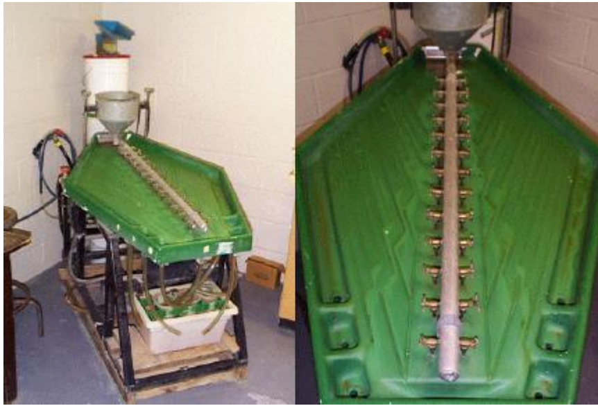
Figura 3.4: Mesa Rogerds utilizada en el Laboratorio de Huellas de Fisión del Union College para la concentración de minerales
