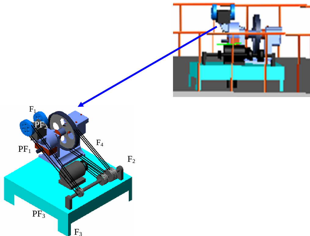
Figura 3.10: Fallas y problemas detectados en el nivel de alimentación y trituración del SASMP. (Tomado y modificado de González, A., y Navarro, W., 2002)
