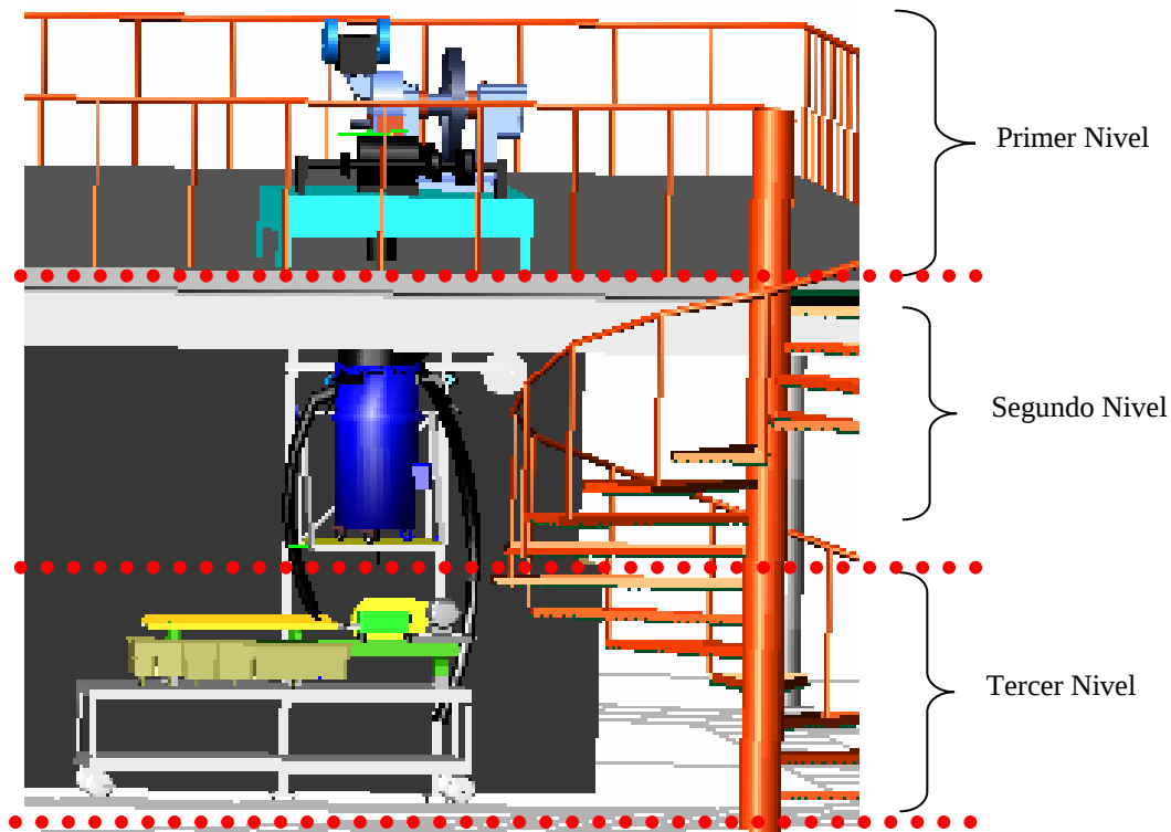
Figura 3.6: Croquis del SASMP, mostrando los tres niveles de funcionamiento.
