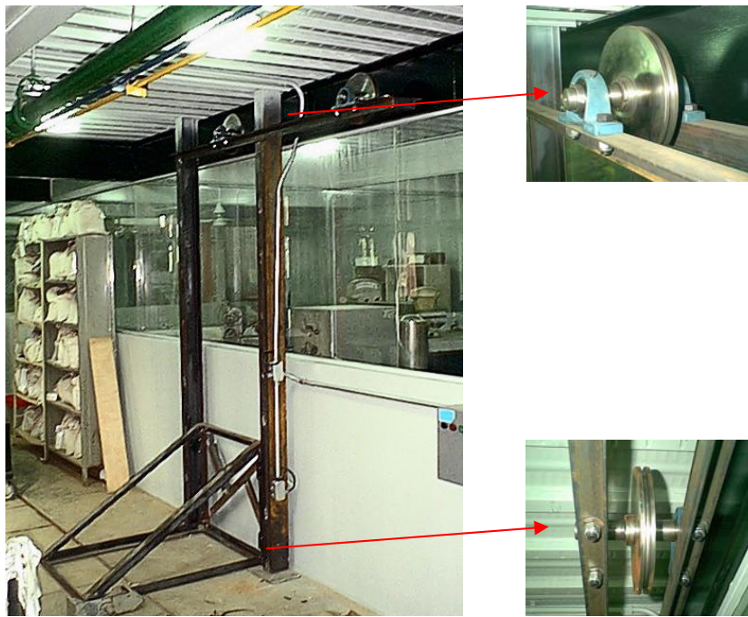
Figura 3.9: Detalles del montacargas construido para el SASMP.
