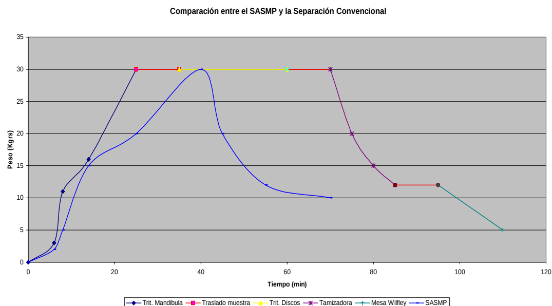
Figura 4.3: Comparación entre el SASMP y el método tradicional de concentración de minerales en condiciones “ideales”.
