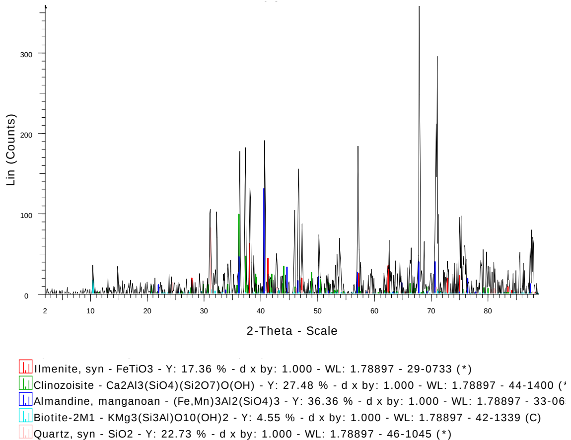
Figura 4.2: Gráfica de la Difracción de rayos X, de la arena estudiada
