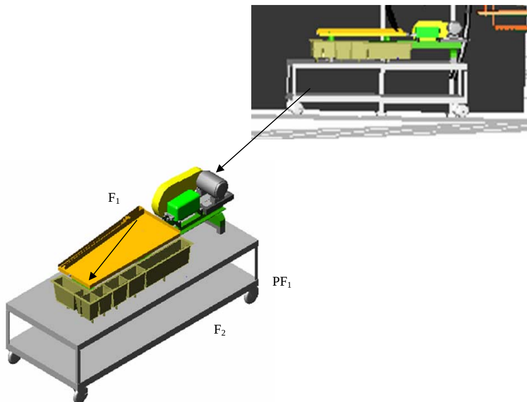
Figura 3.13: Fallas y problemas detectados en el nivel de separación gravimétrica del SASMP. (Tomado y modificado de González, A., y Navarro, W., 2002)
