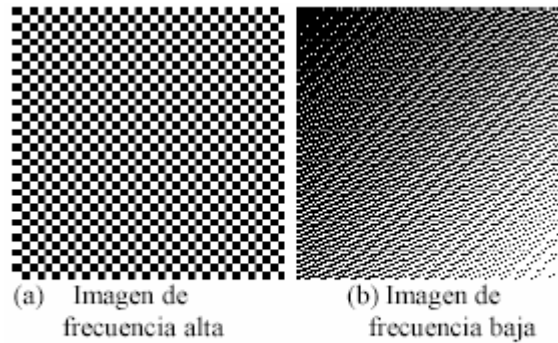
Fig. No. 30 Frecuencias espaciales
