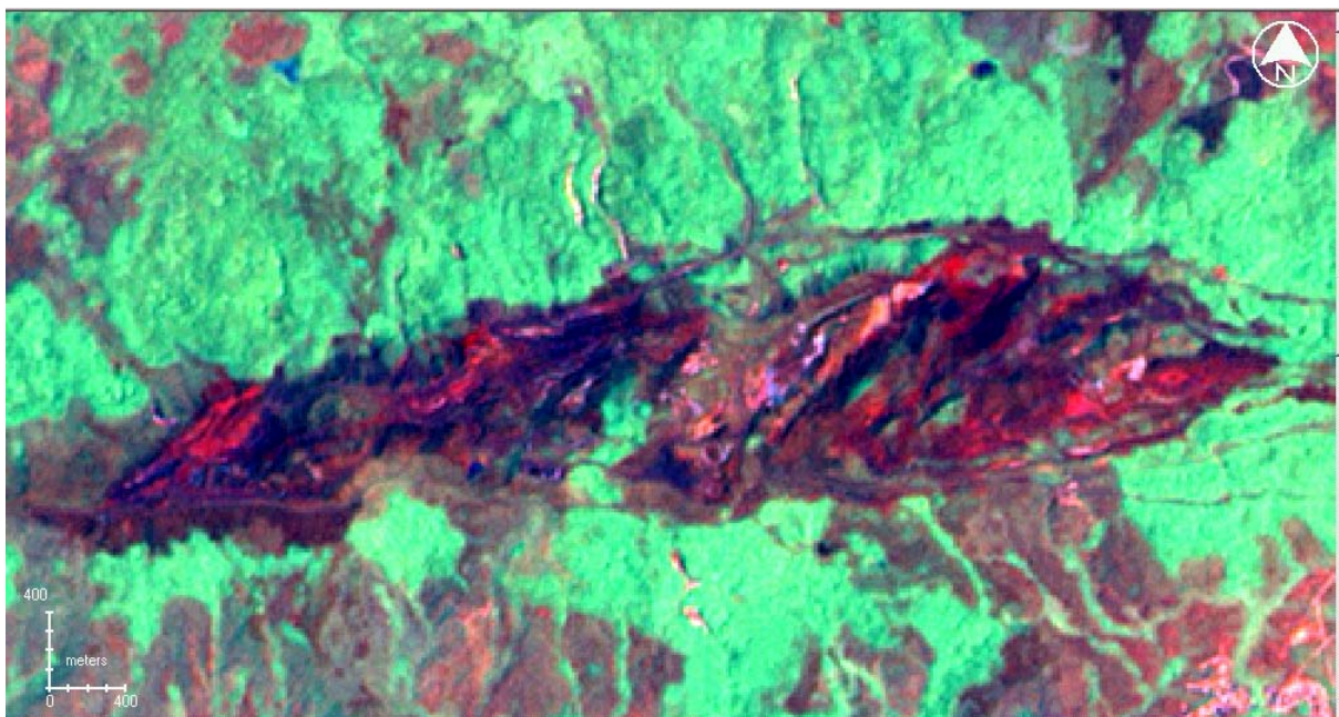
Fig. N° 50a Imagen del Cerro Bolívar combinación de bandas 5-4-2, resultado de la fusión de la imagen multispectral con la Pancromática, obteniéndose así una mejor resolución espacial.
