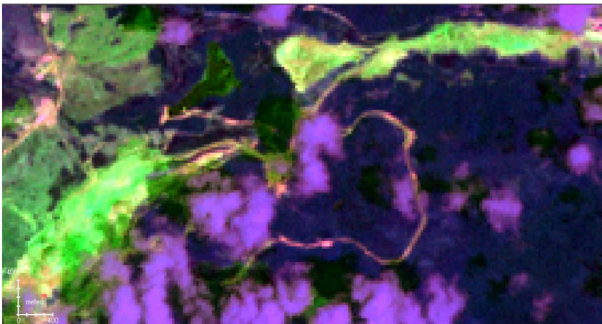
Fig. N° 58b Índice composición mineral del cuadrilátero San Isidro.
