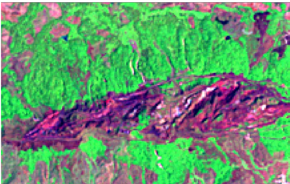
Fig. N° 49: Combinación de las bandas 5-4-2, donde se puede apreciar el realce de colores rojos en el Cerro Bolívar (esquina superior izquierda) y el Cuadrilátero San Isidro (esquina inferior derecha) Escala 1:100.000
