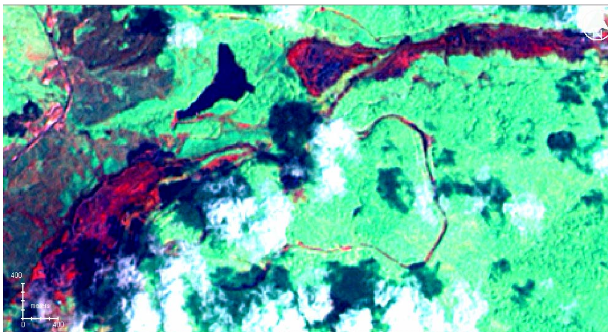
Figura No 50-b Cuadrilátero San Isidro.
