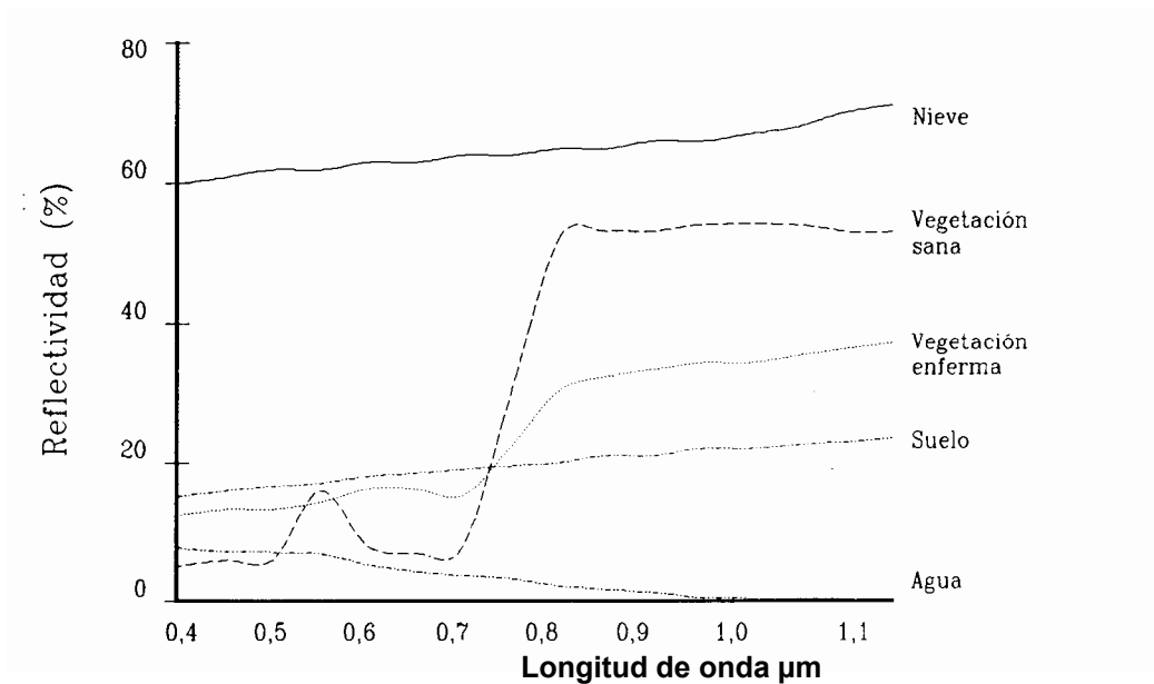
Fig. No.7 Firmas espectrales típicas de distintas cubiertas
