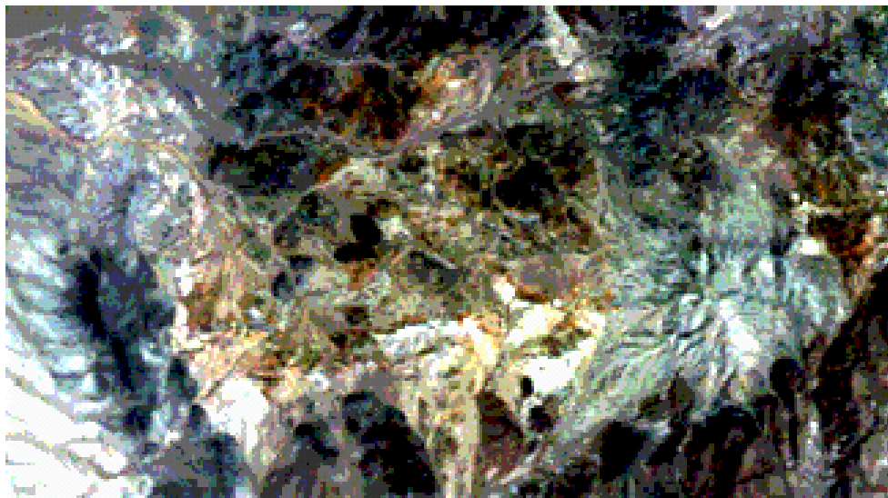
Fig. N° 9 Escena TM del Monte Blanco
