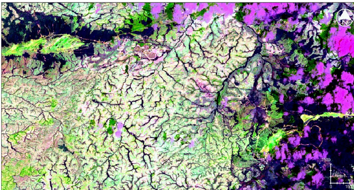
Fig. N° 58 Índice composición mineral, que resalta principalmente en verde la presencia de minerales ferrosos.
