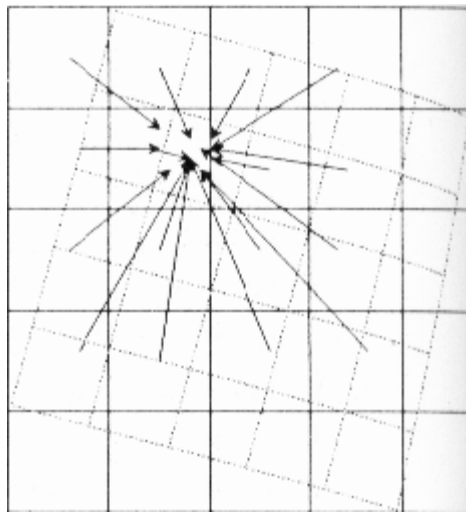
Fig. Nº 23 Efecto del algoritmo de transferencia de Convolución cúbica en la corrección geométrica de la imagen
