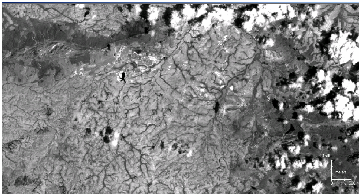
Fig. N° 57 Cociente de bandas para realce de minerales arcillosos (tonos blancos) Escala 1:100.000
