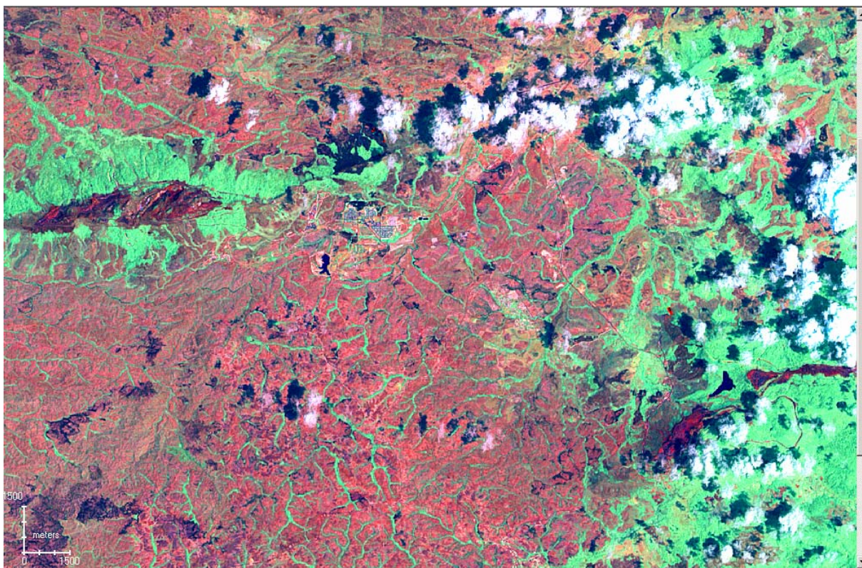
Fig. N° .50 Resultado de la fusión entre la imagen multiespectral y pancromática combinación de bandas 5-4-2
