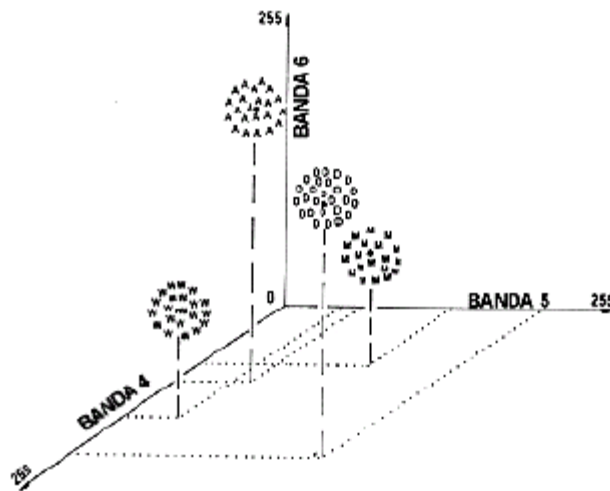
Fig. N° 31 Agrupaciones (cluster) en la clasificación no supervisada
