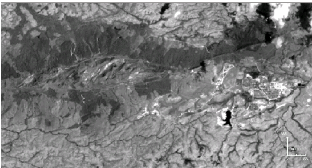
Fig. N° 57a Cociente de bandas para realce de minerales arcillosos del Cerro Bolívar y sus adyacencias. Se puede observar en tonos blancos poca presencia de minerales arcillosos en el Cerro Bolívar Escala 1:50.000
