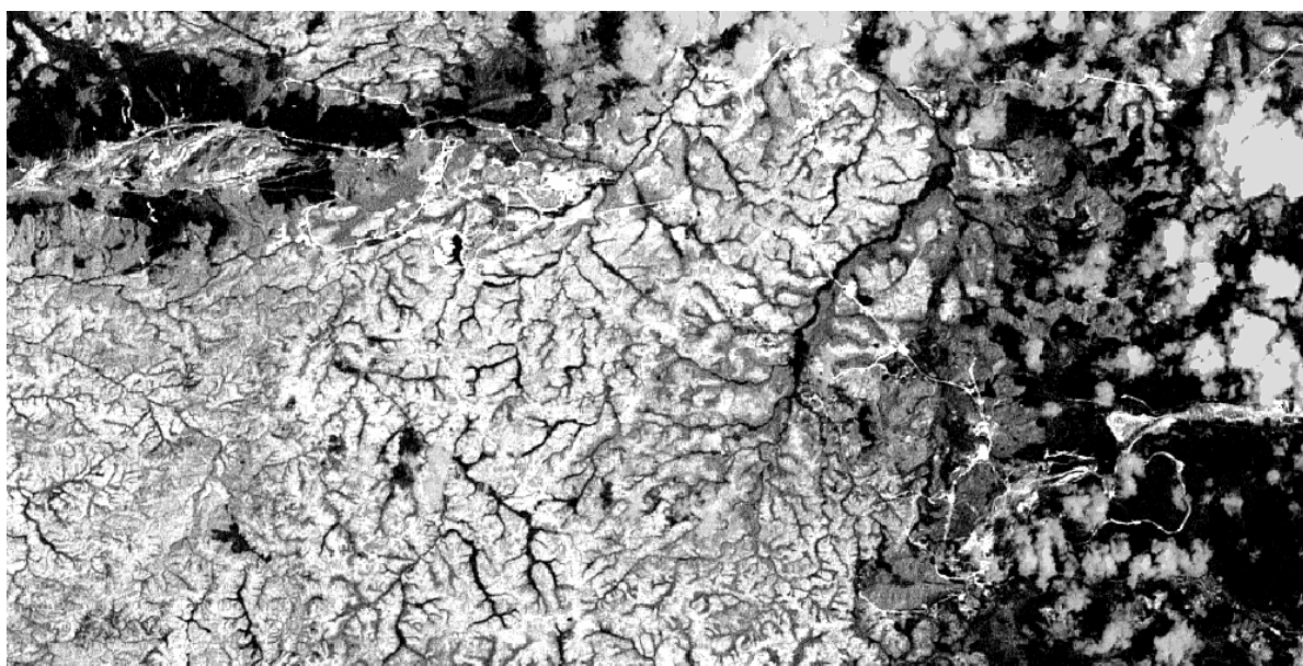
Fig. N° 55 Cocientes de bandas para resaltar óxidos de hierro (tonos más blancos)
