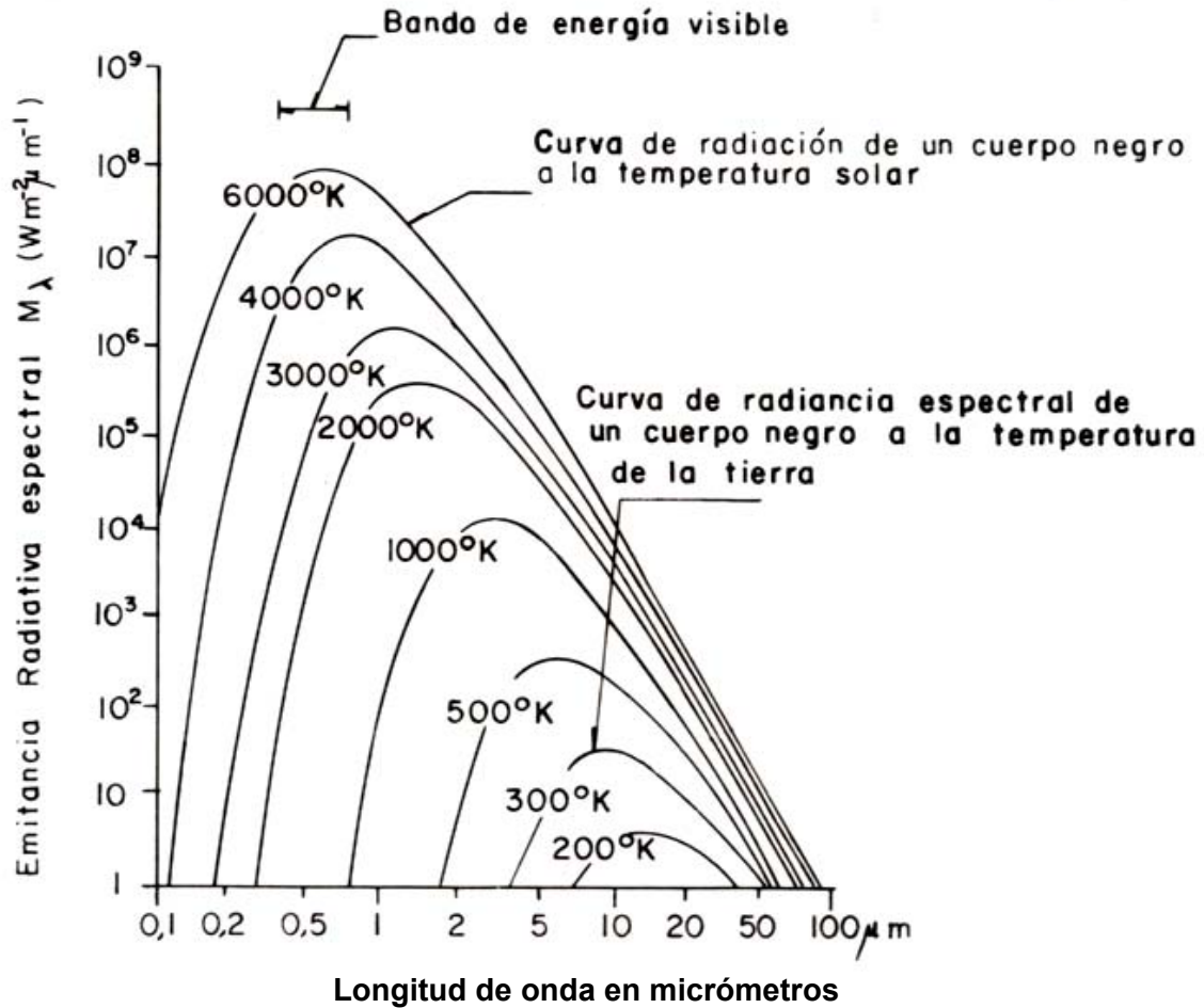
Fig. No. 4 Curva de emitancia radiativa
