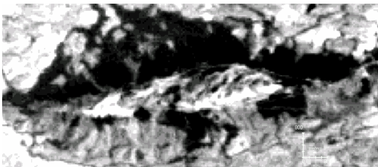
Fig. N° 54a Imagen del Cerro Bolívar banda 6 del infrarrojo termal, en donde se observan varias zonas del Cerro Bolívar con una alta irradiación térmica (zonas blancas) estando estas zonas asociadas a minerales ferrosos principalmente. Las zonas más oscuras de menor irradiancia térmica están asociadas principalmente a vegetación y los tonos grisáceos a zonas de lateritas y minerales arcillosos.
