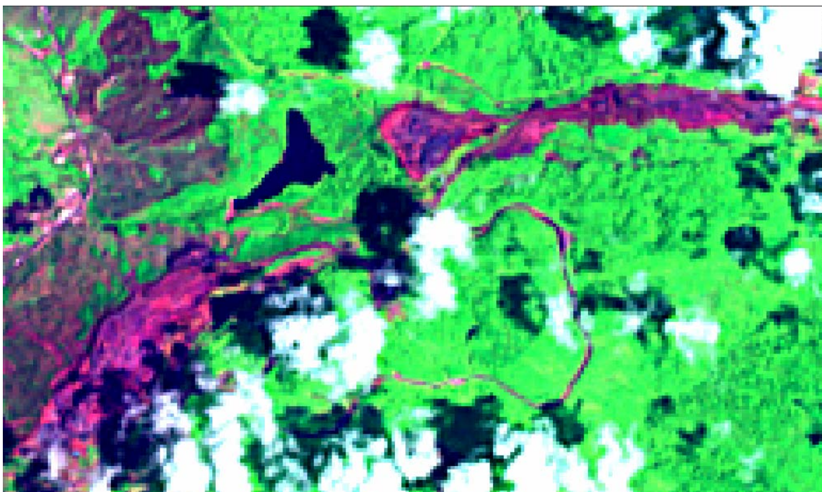
Fig. N° 49-b: Imagen multiespectral Cuadrilátero San Isidro bandas 5-4-2. Aquí también se pueden apreciar como los tonos rojos del Cerro San Isidro (inferior izquierda) y Las Pailas- Los Barrancos (derecha superior) resaltan las zonas de mena de alto tenor, mientras que los tonos azulados resaltan la mena de bajo tenor. Escala 1:25.000
