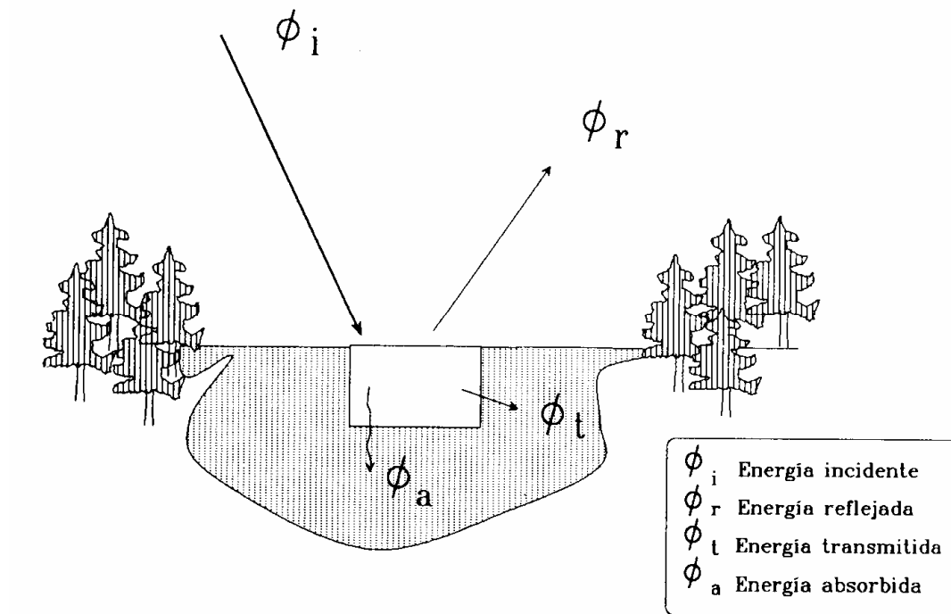
Fig. No. 6 Relación entre flujo incidente y reflejado
