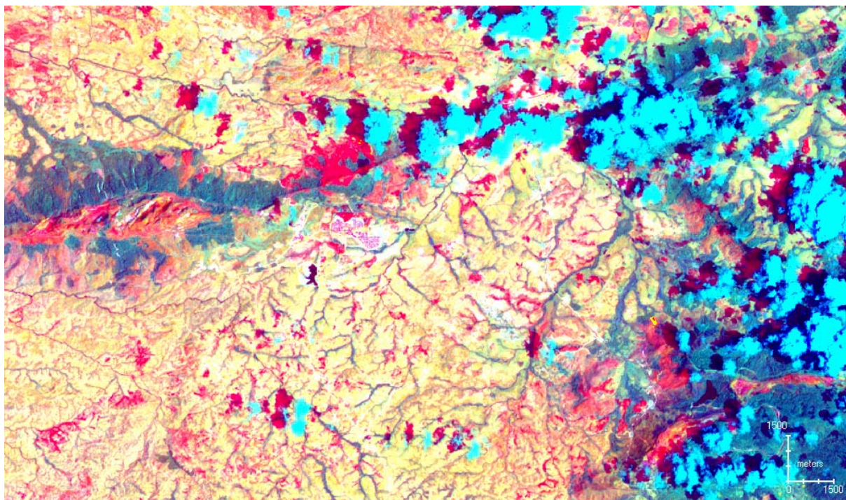
Fig. N° 53. Imagen fusión multiespectral- pancromática combinación de bandas 6-5-3 Escala 1:100.000
