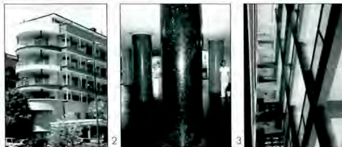
Figura 2 / Detalle de las columnas PB. Hospital Universitario.
