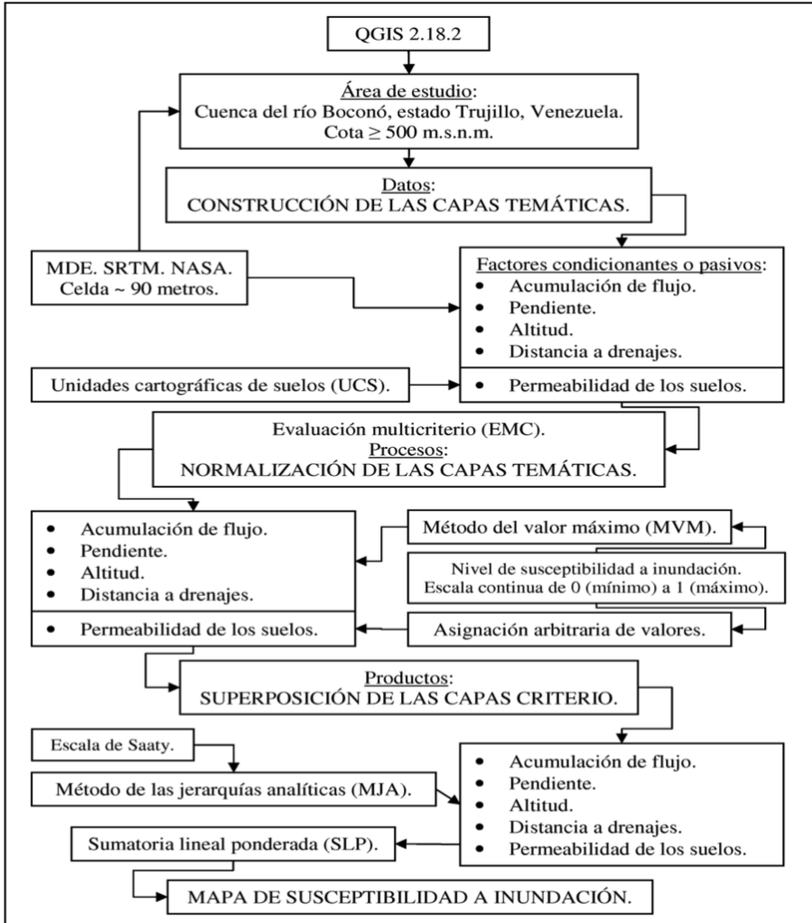
Figura 3. Esquema general metodológico para el desarrollo de la investigación
