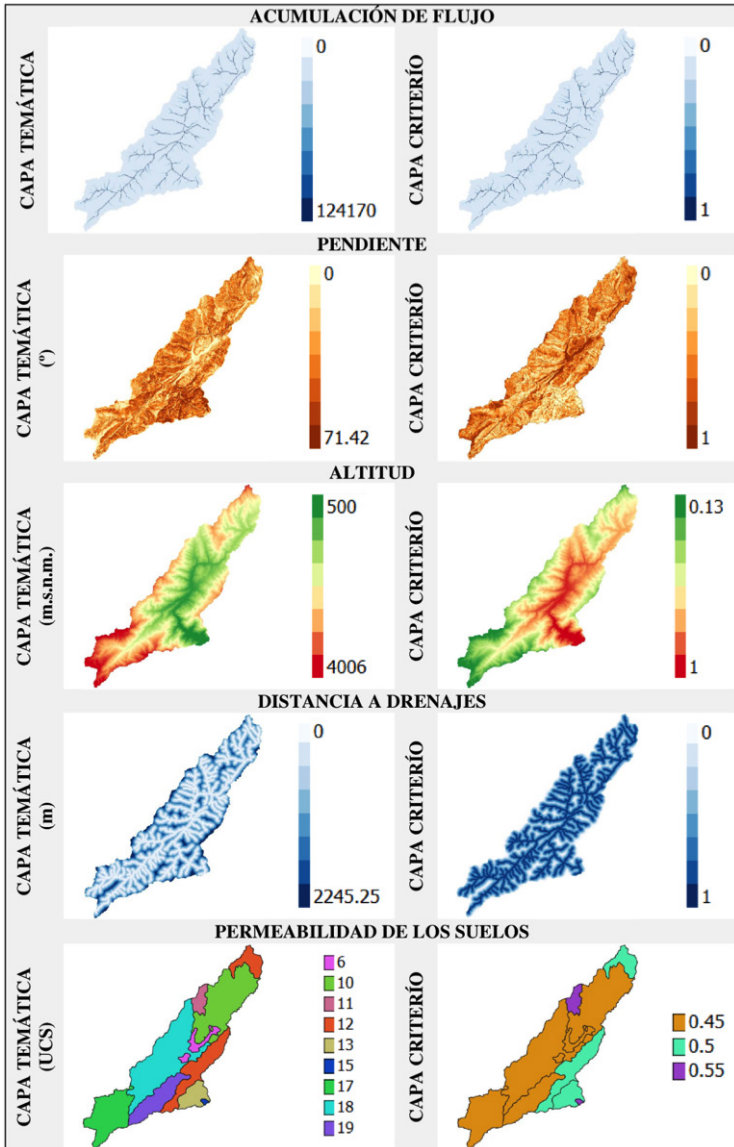
Figura 2. Capas temáticas (generadas) y capas criterio (normalizadas)
