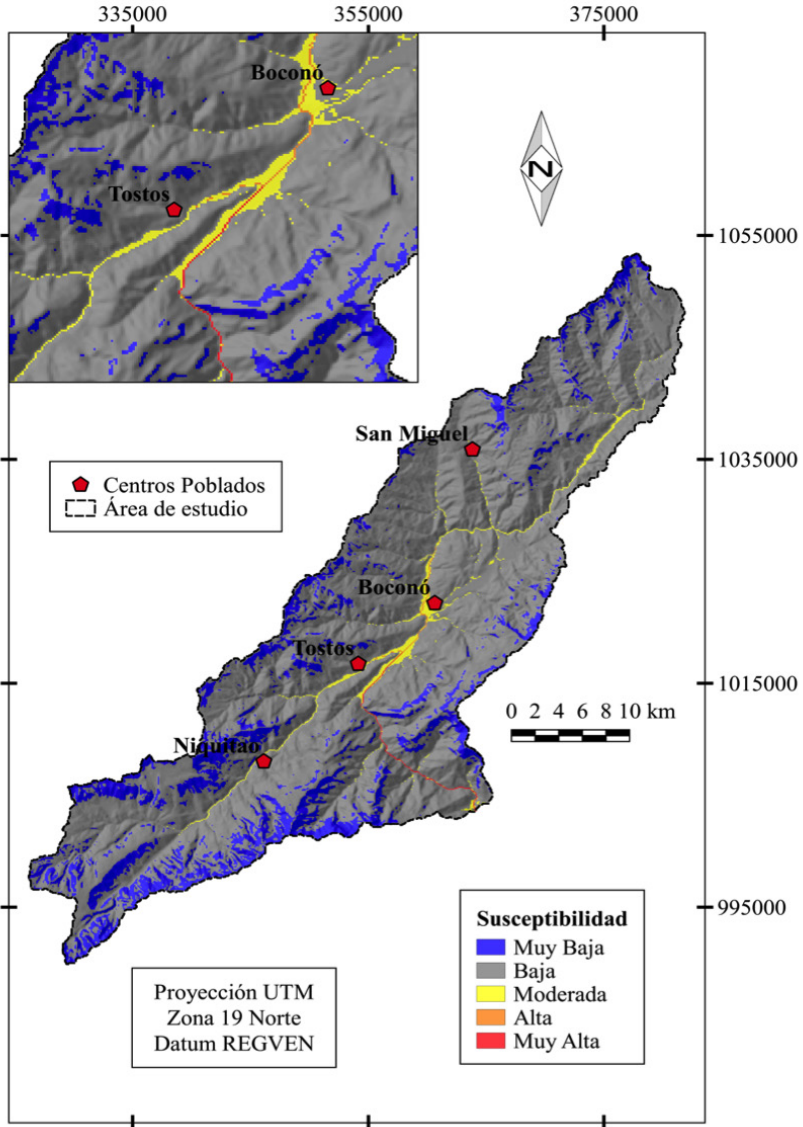
Figura 4. Mapa de Susceptibilidad a Inundación en la cuenca del río Boconó, estado Trujillo, Venezuela
