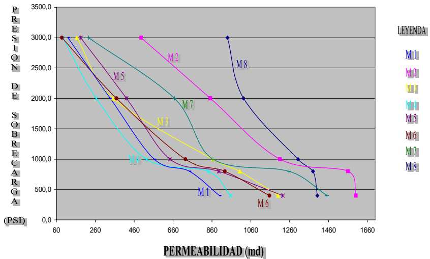
Figura 5. Permeabilidad a diferentes presiones de sobrecarga
