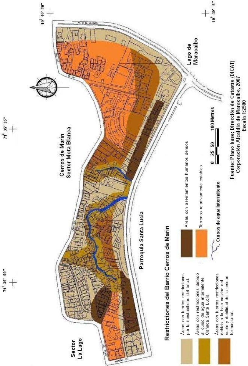
Figura 9. Restricciones de habitabilidad en el Barrio Cerros de Marín, municipio Maracaibo, estado Zulia
