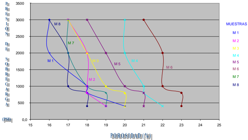
Figura 6. Porosidad a diferentes presiones de sobrecarga
