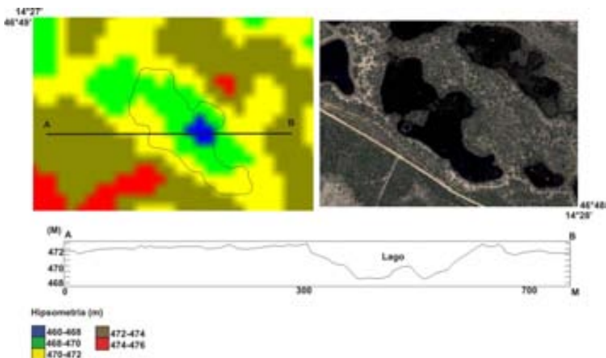
Figura 9. Hipsometria do Lago 4. Município de Alvorada do Norte, estado de Goiás
