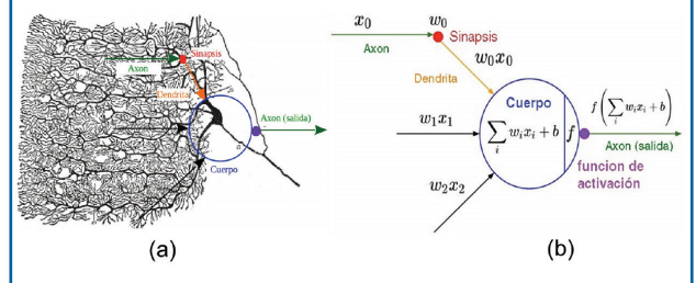
Figura 3. (a) Diagrama que muestra como el funcionamiento y la estructura de las redes neuronales biológicas inspiraron el funcionamiento netamente matemático del primer modelo de neurona artificial, el perceptrón (b).
