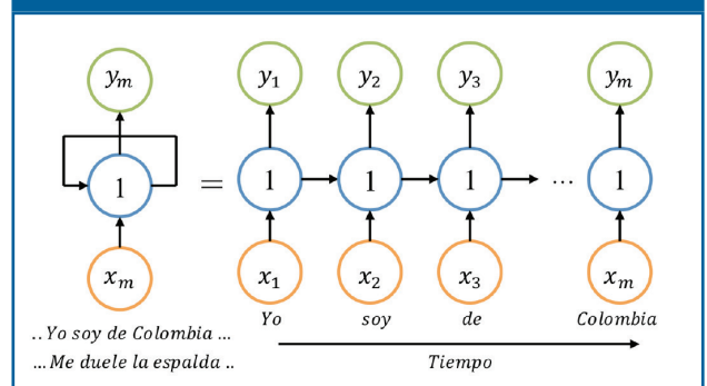
Figura 7. Arquitectura de una Red Neuronal Recurrente
