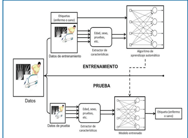
Figura 2. Para reconocer si un paciente tiene cierta enfermedad o no, el ordenador obtiene un conjunto de datos mixtos el cual divide entre datos de entrenamiento y de prueba, una vez el algoritmo seleccionado es entrenado, se evalúa la precisión del modelo al predecir etiquetas de datos de prueba.
