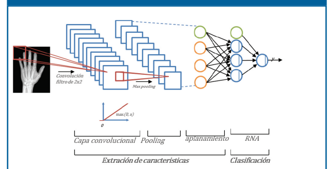
Figura 5. Arquitectura de una Redes Neuronales Convolucionales
