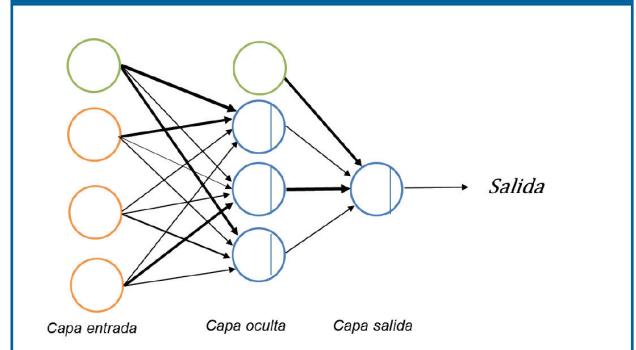
Figura 6. Arquitectura simple de una red neuronal multicapa
