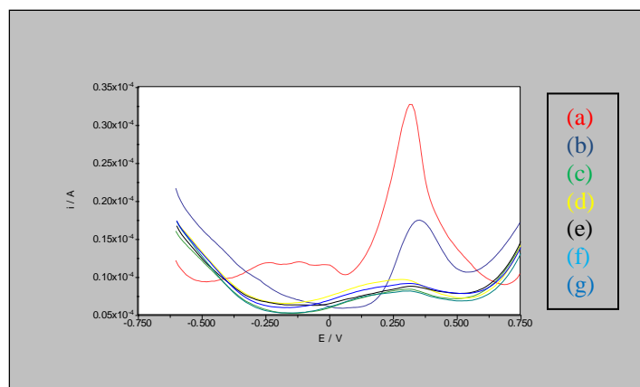
Figura 5. Voltametrías de pulso diferencial en NaH 2 PO 4 /KCl 0,1 M pH 6,20. Para: (a) línea discontinua electrodo Au/TOU, (b) línea discontinua Au/TOU/NaH 2 PO 4 /KCl/Ac 1 hora, (c) línea discontinua Au/TOU/NaH 2 PO 4 /KCl/Ac 1 hora/5mL de E.coli (aprox. 1,5 x10 9 UFC/mL), (d) Au/TOU/NaH 2 PO 4 /KCl/Ac 1 hora/5mL de E.coli (aprox. 1,5 x10 9 UFC/mL) (primer barrido), (e) Au/TOU/ NaH 2 PO 4 /KCl/Ac 1 hora/5mL de E.coli (aprox. 1,5 x10 9 UFC/mL) (segundo barrido) (f) Au/TOU/NaH 2 PO 4 /KCl/Ac 1 hora/5mL de E.coli (aprox. 1,5 x10 9 UFC/mL) (tercer barrido) y (g) Au/TOU/NaH 2 PO 4 /KCl/Ac 1 hora/5mL de E.coli (aprox. 1,5 x10 9 UFC/mL) (cuarto barrido). Ventana de potencial desde -0,6 hasta +0,75mV/s. Atmósfera de N 2 .
