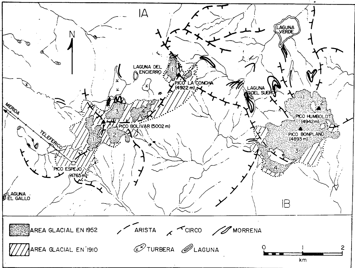
Fig. 1. Extensión de los glaciares en 1910 (Jahn, 1925) y en 1952 (fotografías aéreas, Misión A-34, DCN). Nótese las morrenas neoglaciares, algunas de las cuales fueron depositadas durante la Pequeña Edad de Hielo (siglos XVI a XIX). Los números indican los glaciares de la Tabla 1.
