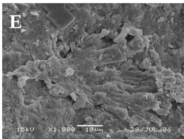
Fig. 7e. Imagen MEB una superficie rota, donde se nota una distribución aproximadamente radial de los cristales de aheylita.
