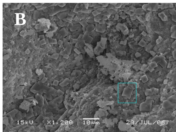
Fig. 7a,b. Imágenes de microscopio electrónico de barrido (MEB) de la superficie de una esfera de aheylita. El recuadro de arriba ubica a la Fig. 8b y el de abajo a la Fig. 8a.
