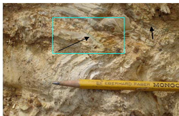
Fig. 5. Detalles de la ocurrencia de aheylita. Cerca de la punta del lápiz se observa un pequeño pliegue de arrastre. Abajo ampliación del área del recuadro azul.
