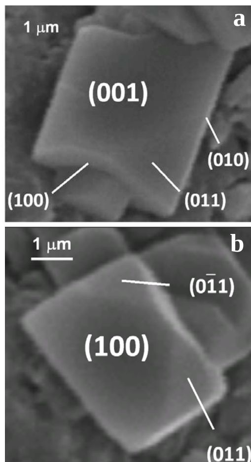
Fig. 8. Combinación de varias formas pinacoidales que conforman los cristallitos de aheylita. a) Formas pinacoidales a: {100}, b: {010} y c: {001}, combinadas con un pinacoide {011} que genera una faceta triangular muy prominente. b) Forma pinacoidal a: {100} combinada con dos formas conjugadas {011} y {011} que generan dos facetas triangulares prominentes en la parte derecha del cristallito.
