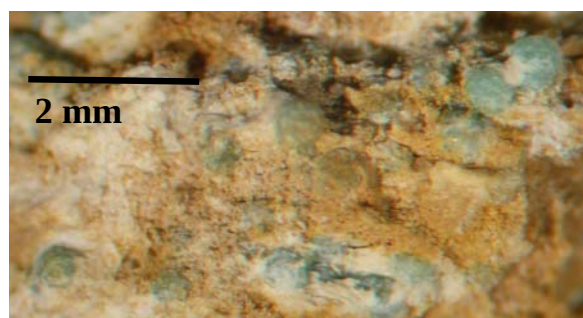
Fig. 6. Aheylita formando agregados esféricos submilimétricos. Fotografía tomada con lupa binocular.
