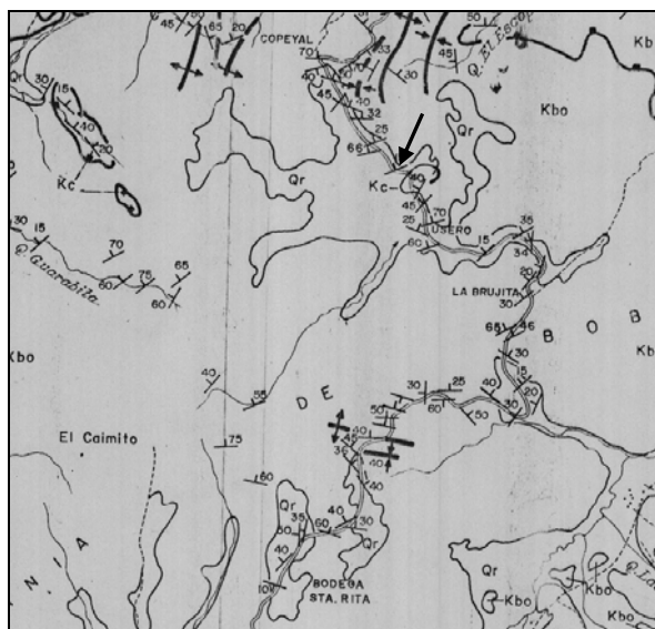
Fig. 3. Fragmento del mapa geológico de BELLIZZIA & RODRÍGUEZ (1969). Kbo: Formación Bobare, Kc: Formación Carorita, Kb: Formación Barquisimeto. Este mapa abarca la misma zona y esta a la misma escala de la figura anterior.
