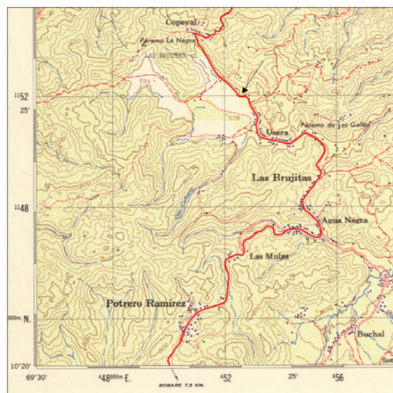
Fig. 2. Mapa de ubicación del afloramiento estudiado (flecha). Fragmento de la hoja 6347, Aguada Grande, D.C.N., 1969.
