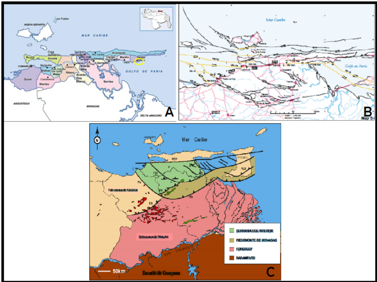
Fig. 1. a) Área de trabajo, localidad de Güiría. b) Mapa de fallas Cuaternarias en el Oriente de Venezuela. En el mapa se refleja la diversidad de fallas presente en el país (AUDEMARD et al. 2000). c) Principales elementos estructurales de la Cuenca Oriental de Venezuela. A breviaturas: FEP= Falla El Pilar; FSF= Falla San Francisco; FP= Falla Pirital; FU= Falla de Urica; FLB= Falla Los Bajos; FD= Frente de deformación (Tomado de HUNG 1997).
