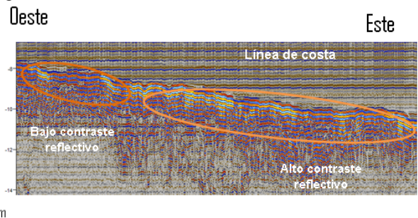
Fig. 7. Sección sísmica longitudinal #002. Se muestra un cambio en los coeficientes de reflexión en sentido oeste – este, suponiendo cambios de materiales de arcillosos a más arenosos en el mismo sentido.
