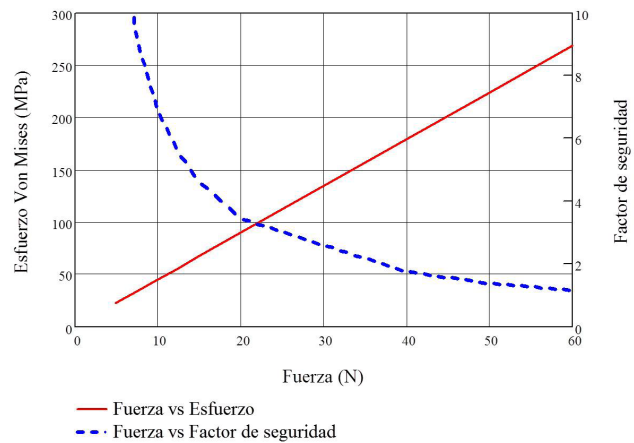
Figura 7. Fuerza de tracción aplicada vs. esfuerzo de von Mises y factor de seguridad en el modelo analizado
