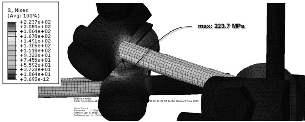
Figura 9. Detalle de la distribución de esfuerzos de Von Mises en la zona crítica
