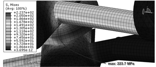
Figura 12. Detalle de concentración de esfuerzos en la barra
