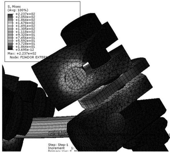
Figura 10. Detalle de la distribución de esfuerzos de von Mises en la sección transversal en la zona crítica
