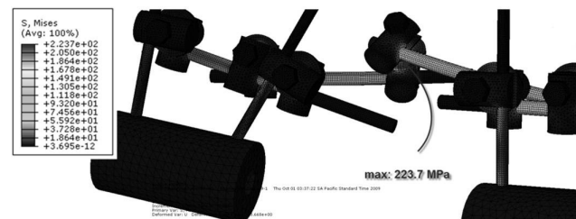
Figura 8. Distribución de esfuerzos de Von Mises para una fuerza de tracción de 50 N
