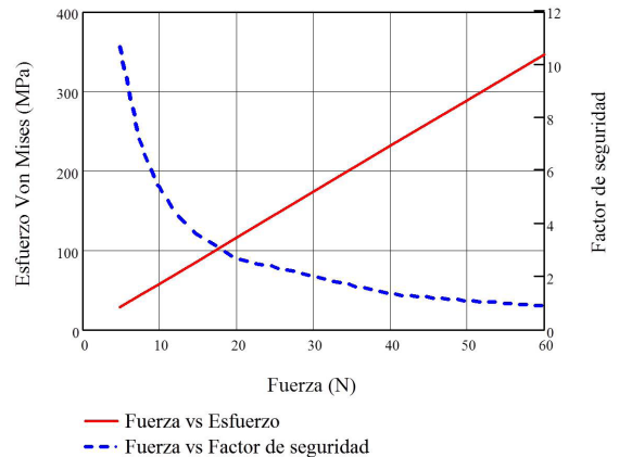
Figura 13. Fuerza de flexión aplicada vs. esfuerzo de von Mises y factor de seguridad en el modelo analizado
