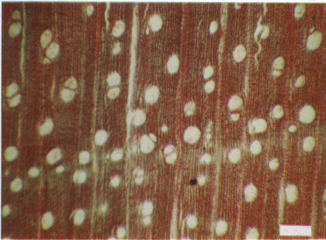
Fig. 10. M. quadrangularis : Poros solitarios, múltiples radiales de 2-3, abundantes tílides (Barra = 100 \mu m).
