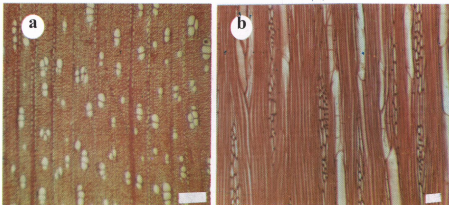
Fig. 8. L. neriifolius : a. Poros solitarios, múltiples radiales de 2-3 (Barra = 300 \mu m). b. Radios menores de 1 mm (Barra = 100 \mu m).
