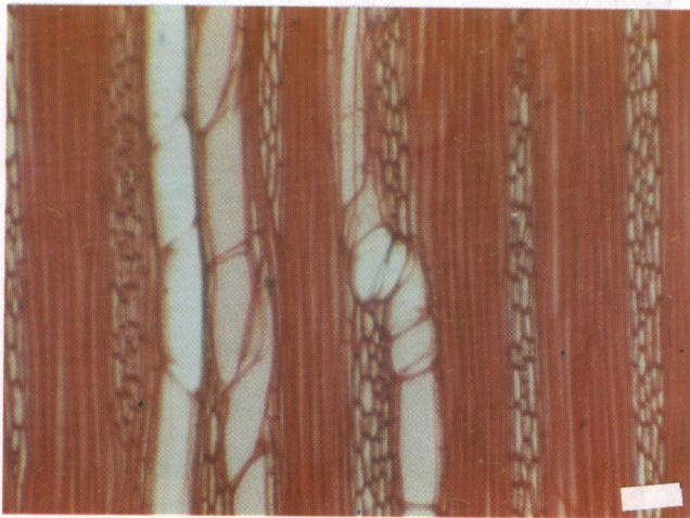
Fig. 5. C. tachirensis : Radios hasta de 5 células de ancho; vaso interceptado por radio (Barra = 100 \mu m).
