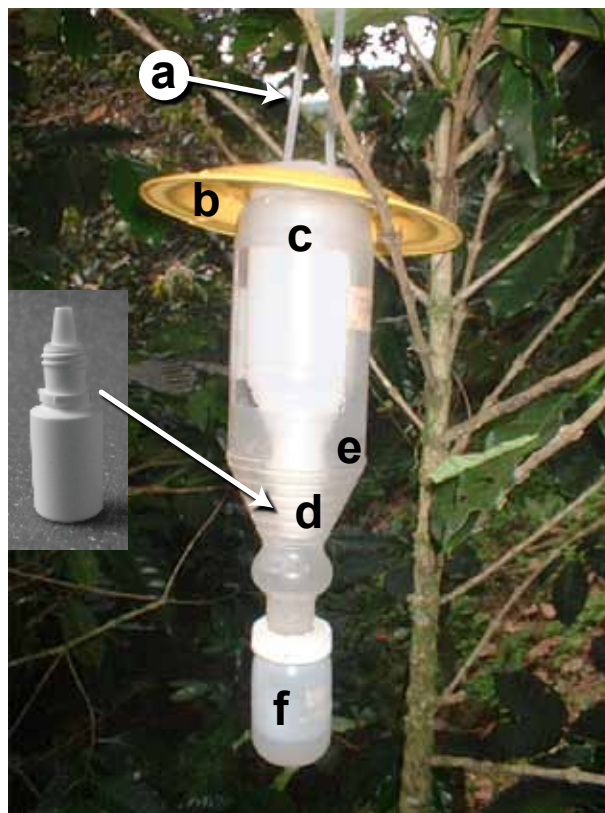
Figura 1. Trampa de interceptación Yessica (Desarrollo Tecnológico de Eutimio González). Componentes: a) dispositivo suspensor, b) pluvioprotector, c) cilindro interceptor, d) dispensador tipo gotero ( \varnothing=2 mm) para emisión de volátiles ( 150\mu\text{L/d} ) provisto con metanol-etanol 3:1 y articulado en el interior del cuello del cilindro interceptor, e) cilindro externo con embudo para desplazamiento en caída libre f) frasco colector con agua
