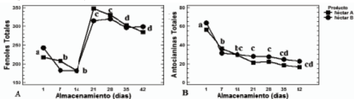
FIGURA 1. A. Fenoles totales durante almacenamiento. B. Antocianinas totales durante almacenamiento. Los datos se presentan como el promedio \pm desviación estándar. Las letras distintas indican diferencias estadísticamente significativas, según la prueba de Tukey ( P < 0,05 ).
