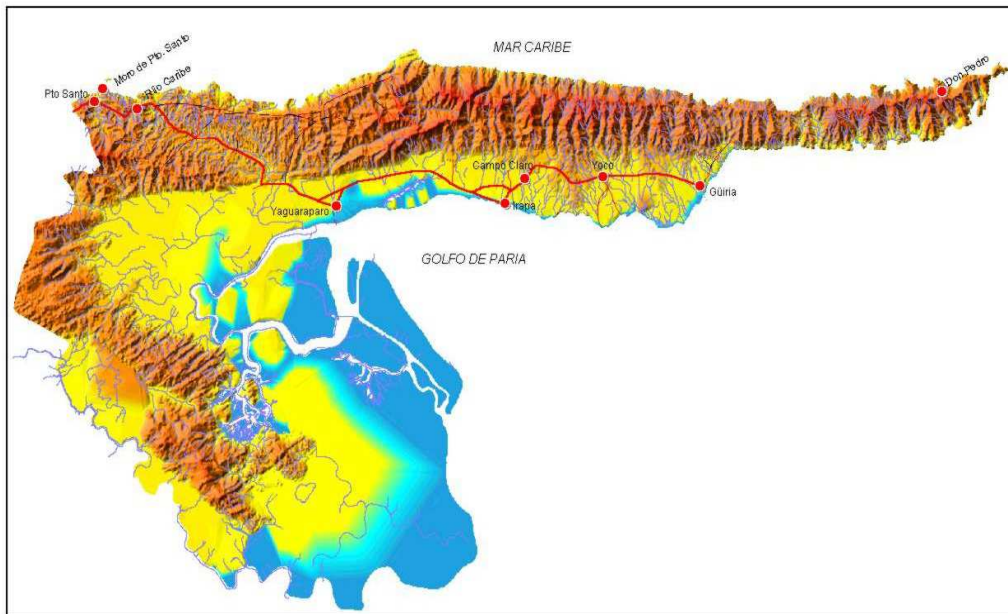
Figura 3. Sobreposición de coberturas de hidrografía, vialidad y centros poblados sobre Modelo Digital de Terreno, mostrando flujos de drenaje.
