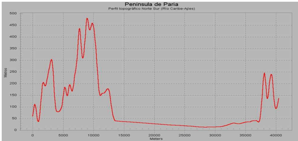
Figura 2. Península de Paria. Perfil topográfico Norte-Sur mostrando las diferentes alturas.
