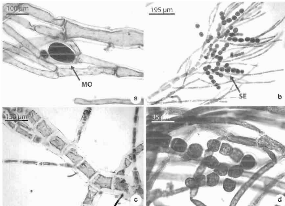
Figura 4 – a. Monosporus indicus – ramas con monosporangios (MO). b-d. Seirospora occidentalis – b. porción distal mostrando seiosporangios (SE); c. detalle de la porción basal; d. detalle de la cadena de seiosporangios.
