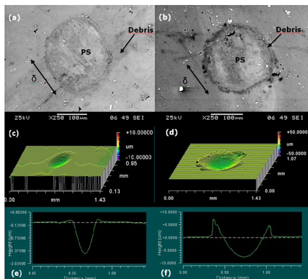
Figura 9. Fotomicrográficas por MEB y perfilometrías de la aleación 7075-T6 ensayada a una carga normal aplicada de 25 N, \delta = 50 \mu\text{m} : (a) y (b) Morfologías de las huellas de desgaste de sustrato a 10^4 y 10^5 ciclos. (c) y (d) Perfiles 3D del sustrato a 10^4 y 10^5 ciclos. (e) y (f) Perfiles 2D del sustrato a 10^4 y 10^5 ciclos.
