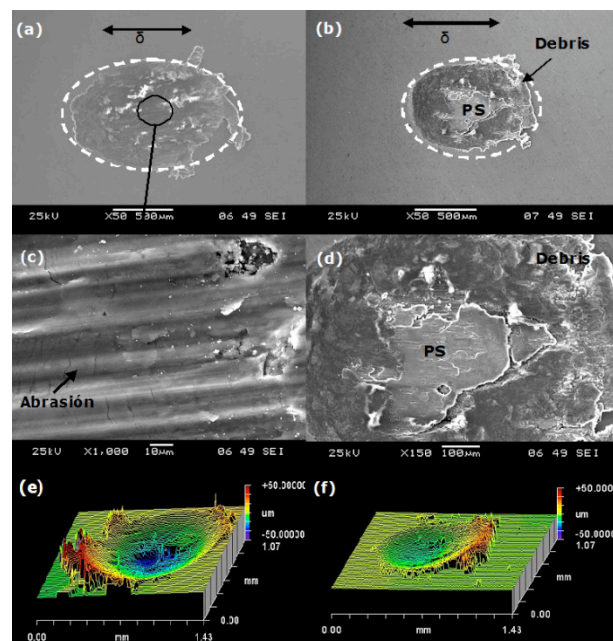
Figura 10. Fotomicrográficas por MEB y perfilometrías de AA 7075-T6 ensayada a una carga normal aplicada de 75 N, \delta = 250 \mu\text{m} : (a) y (b) Morfologías de las huellas de desgaste de sustrato a 10^4 y 10^5 ciclos. (c) Vista detallada del área indicada en (a). (d) Morfología de la huella de desgaste del sustrato a 10^5 ciclos, a una magnificación de 150x. (e) y (f) Perfiles 3D del sustrato a 10^4 y 10^5 ciclos.
