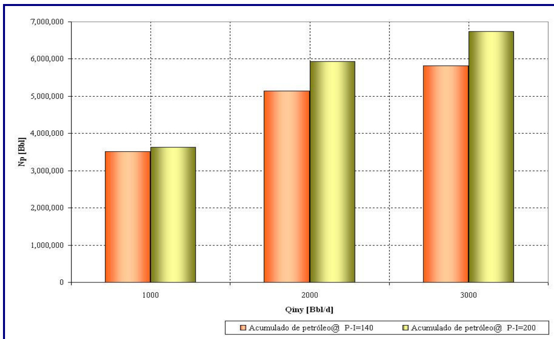
Figura A- 5: Gráfico de sensibilidad de espaciamiento para diversas tasas de inyección, con una sección horizontal de los pozos productores de 320m. (4prodH_2icvH)
