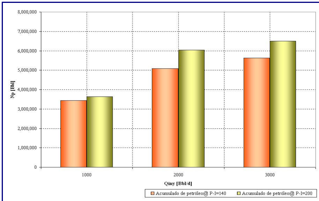
Figura A- 4: Gráfico de sensibilidad de espaciamiento para diversas tasas de inyección, con una sección horizontal de los pozos productores de 200m. (4prodH_2icvH)
