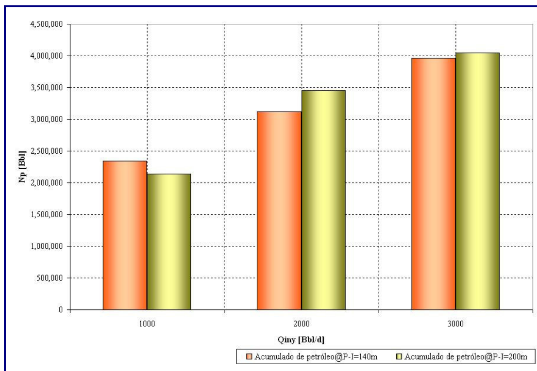
Figura A- 1: Gráfico de sensibilidad de espaciamiento para diversas tasas de inyección, con una sección horizontal de los pozos productores de 200m. (2prodH_1icvH)
