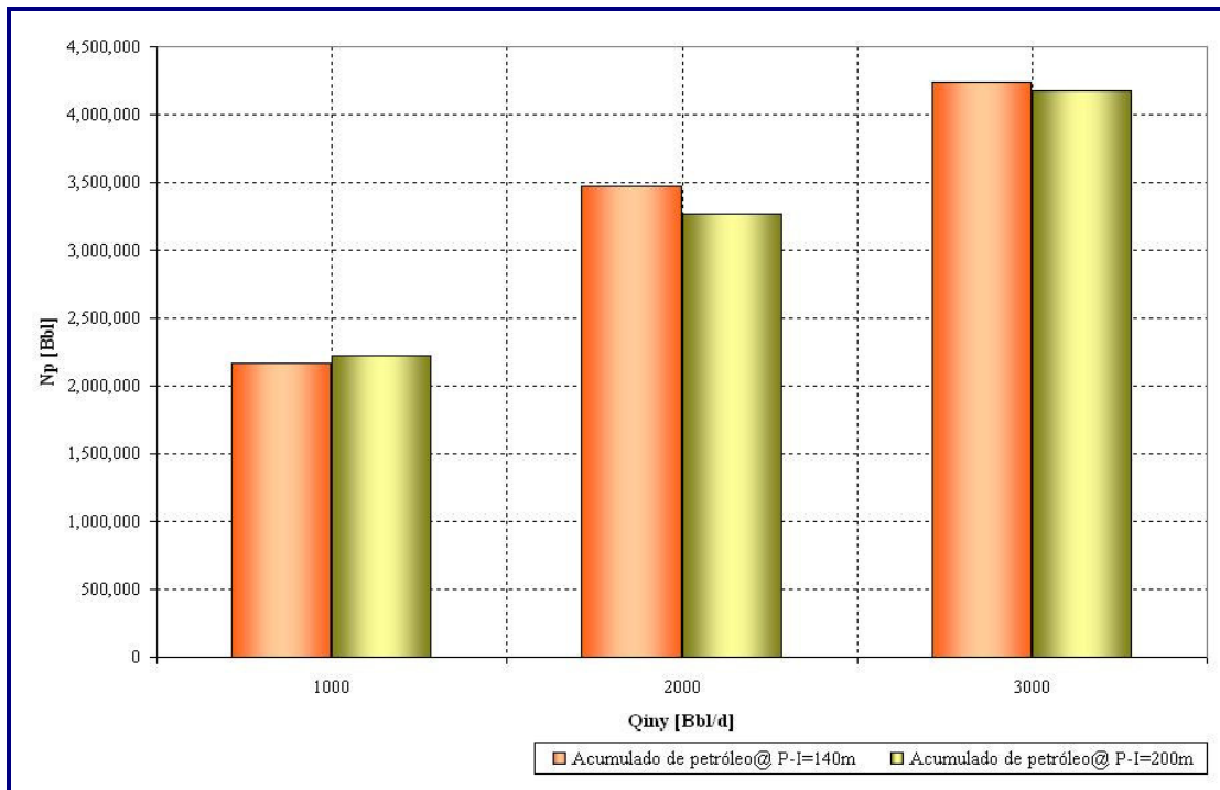
Figura A- 3: Gráfico de sensibilidad de espaciamiento para diversas tasas de inyección, con una sección horizontal de los pozos productores de 500m. (2prodH_1icvH)
