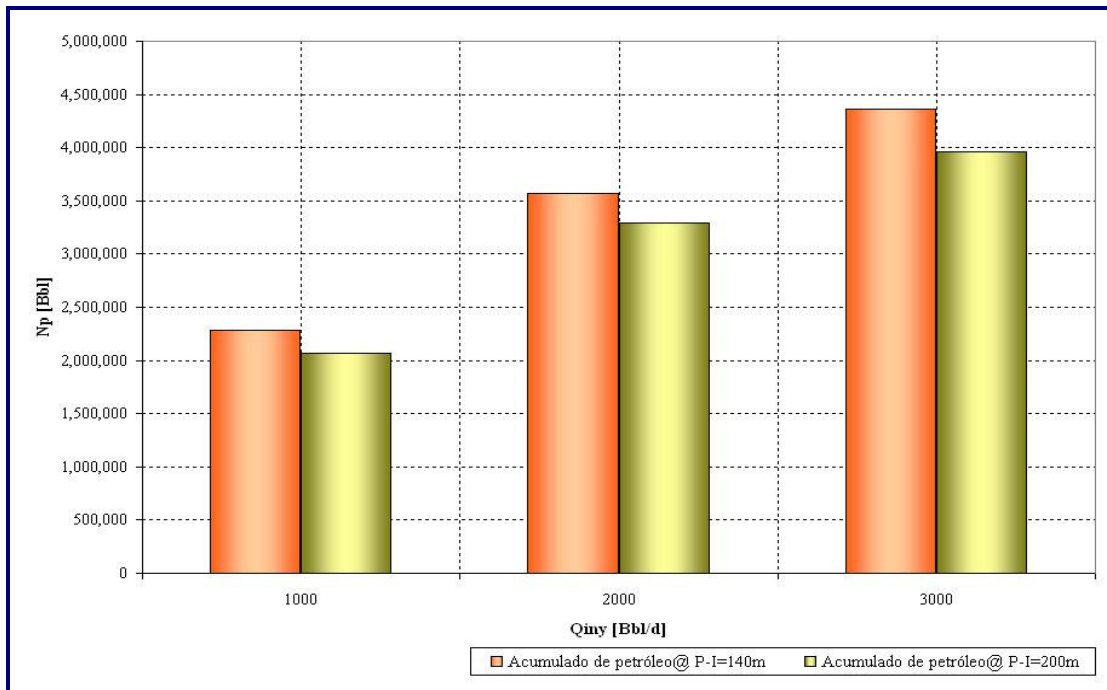
Figura A- 2: Gráfico de sensibilidad de espaciamiento para diversas tasas de inyección, con una sección horizontal de los pozos productores de 320m. (2prodH_1icvH)
