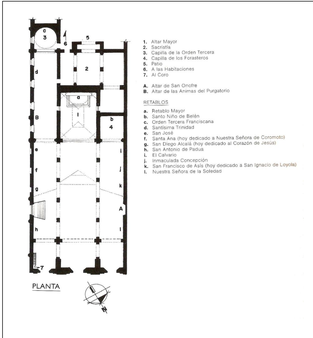
Fig. 5. Estado actual de la iglesia San Francisco
