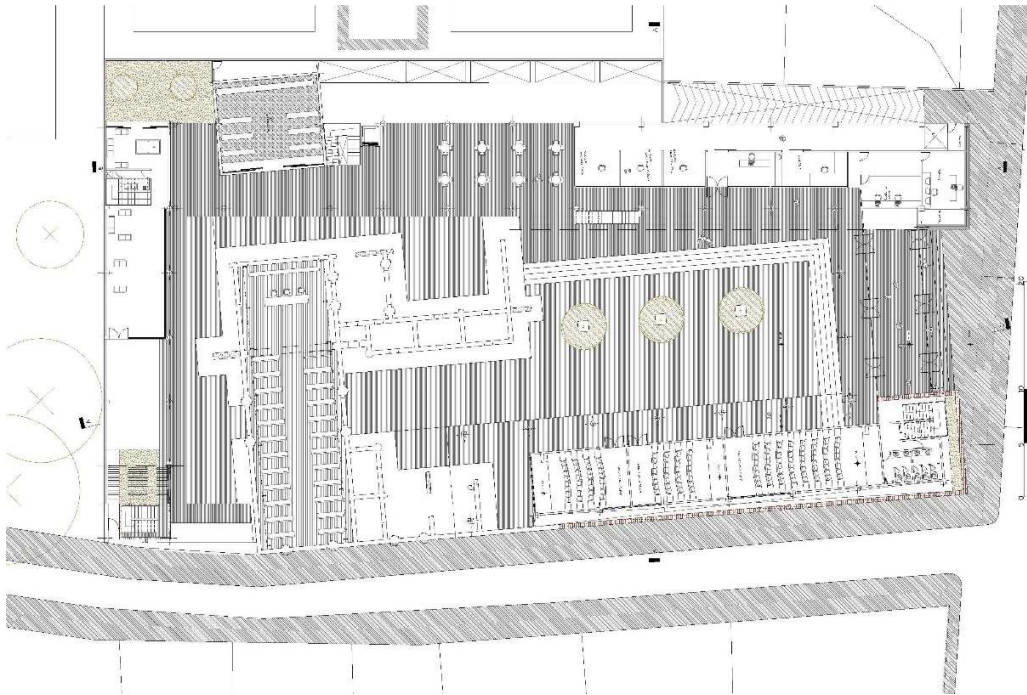
Figura 1: Planta baja
