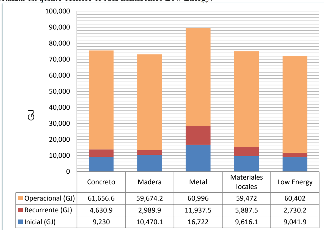
Figura 4: Gráfico de energía consumida durante el ciclo de vida del edificio
