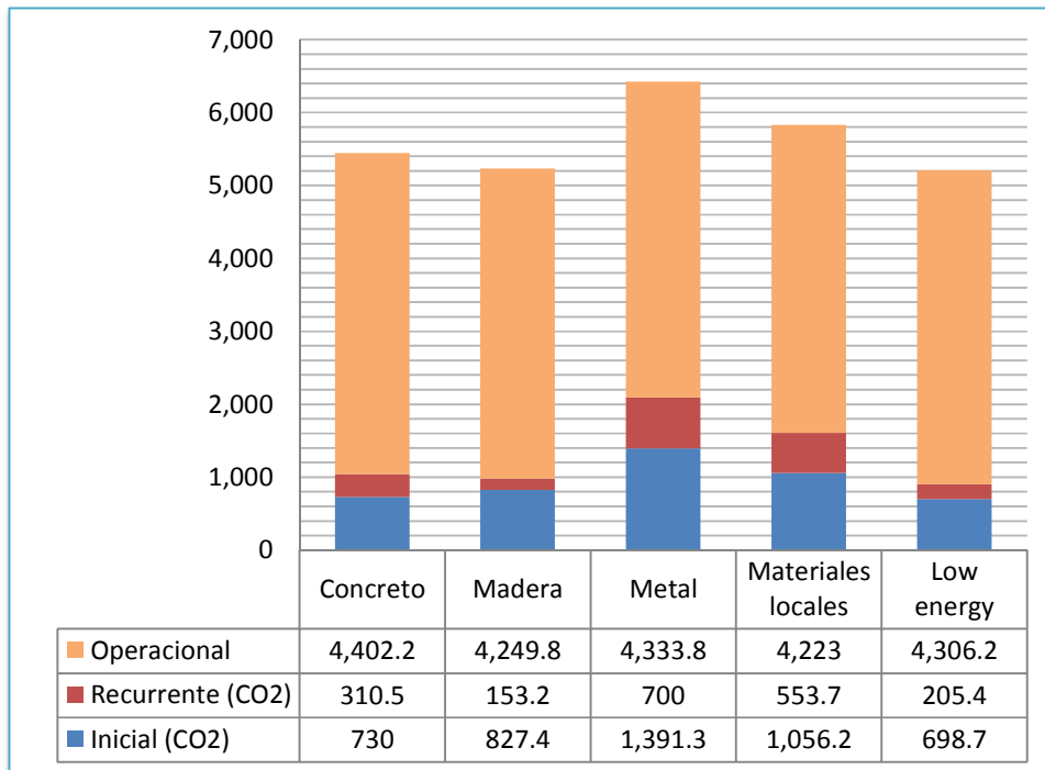
Figura 5: Gráfico de emisiones de CO 2 durante el ciclo de vida del edificio
