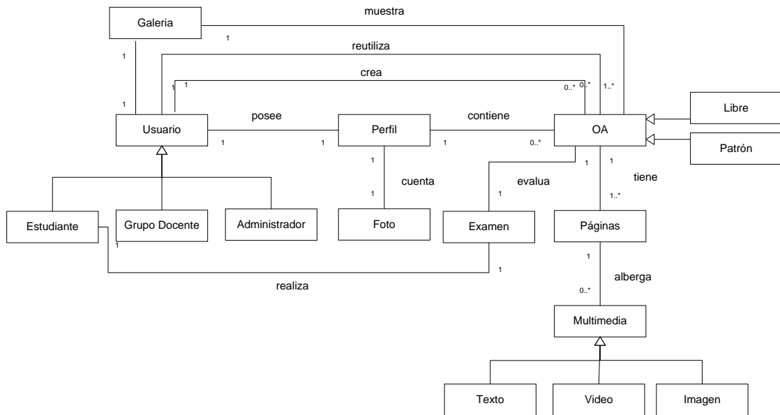
Figura 8. Modelo de Objetos del Dominio
